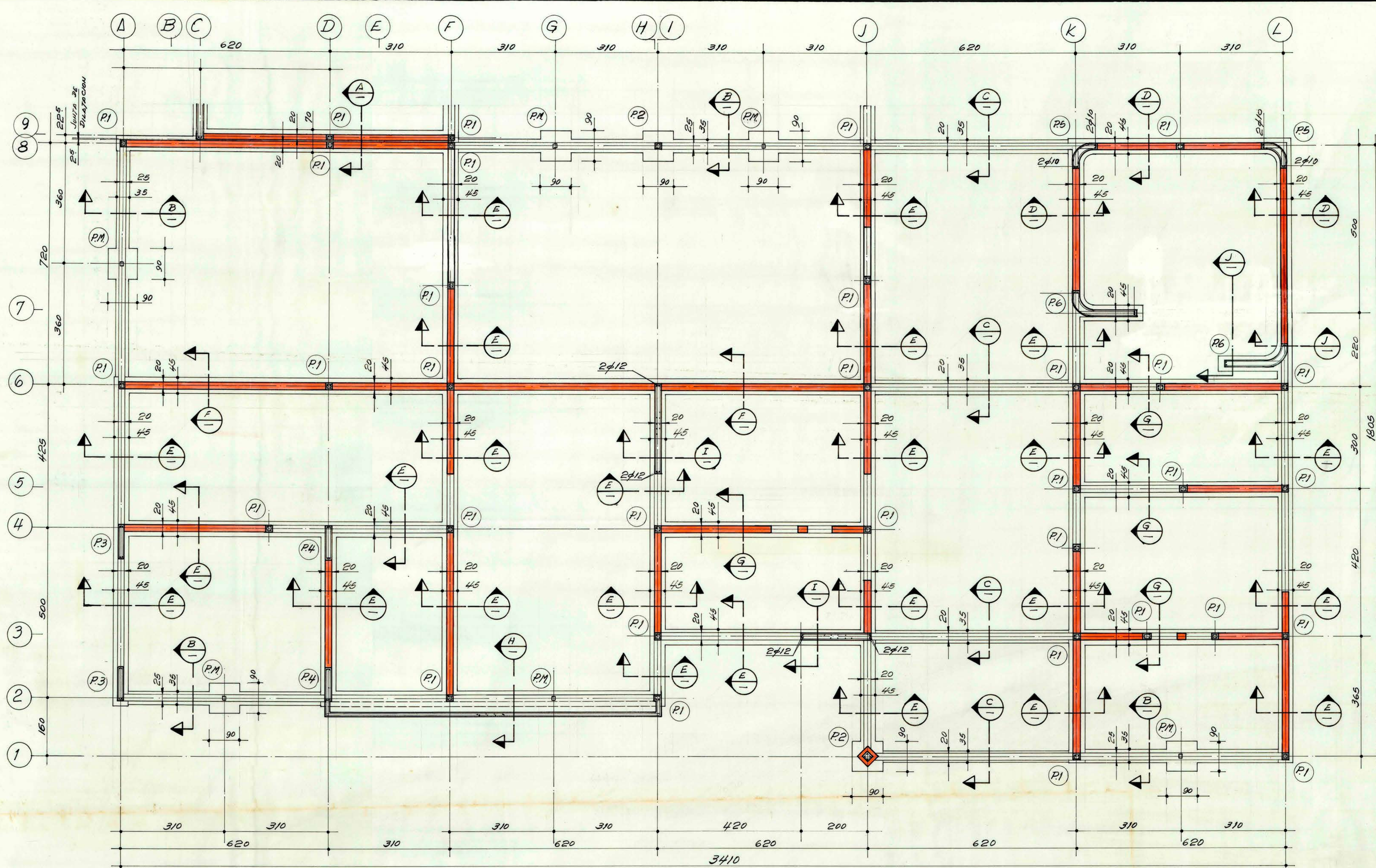
PLANTA DE FUNDACIONES
