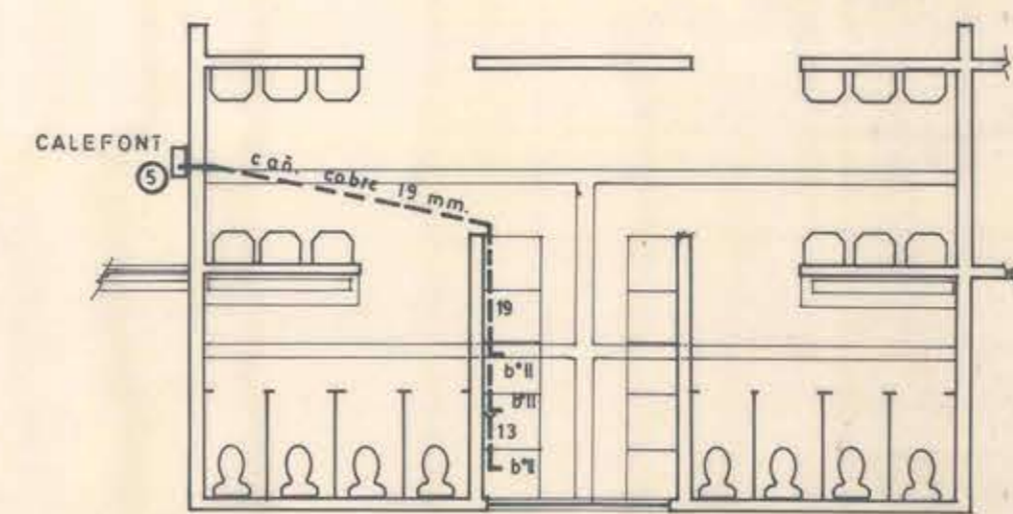
SOLUCIONES AGUA CALIENTE PRIMER PISO ESCALA 1:100
