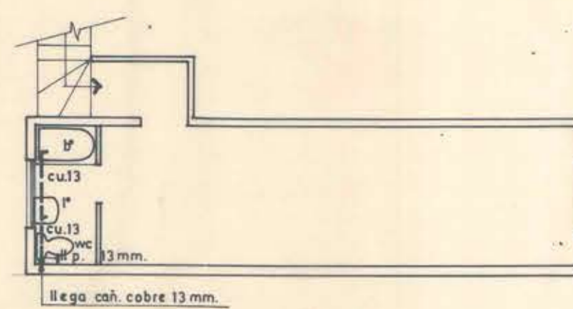
PLANTA 2º PISO AGUA CALIENTE ESCALA 1:100
