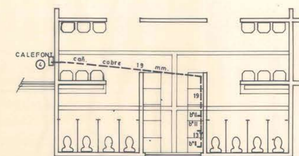
SOLUCIONES AGUA CALIENTE PRIMER PISO ESCALA 1:100
