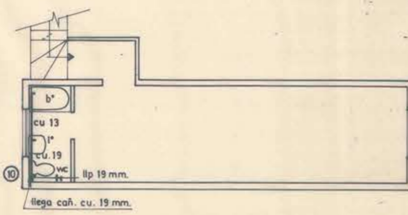
PLANTA 2º PISO AGUA FRIA ESCALA 1:100
