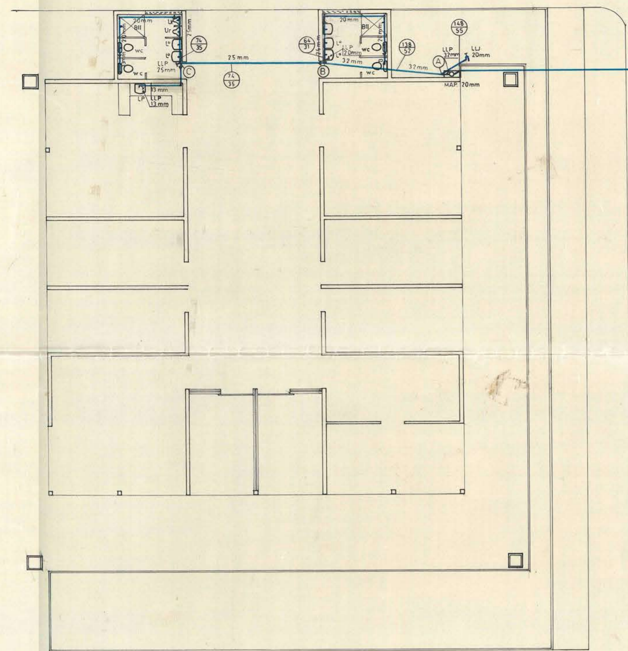
PLANTA AGUA POTABLE Escala 1:100
