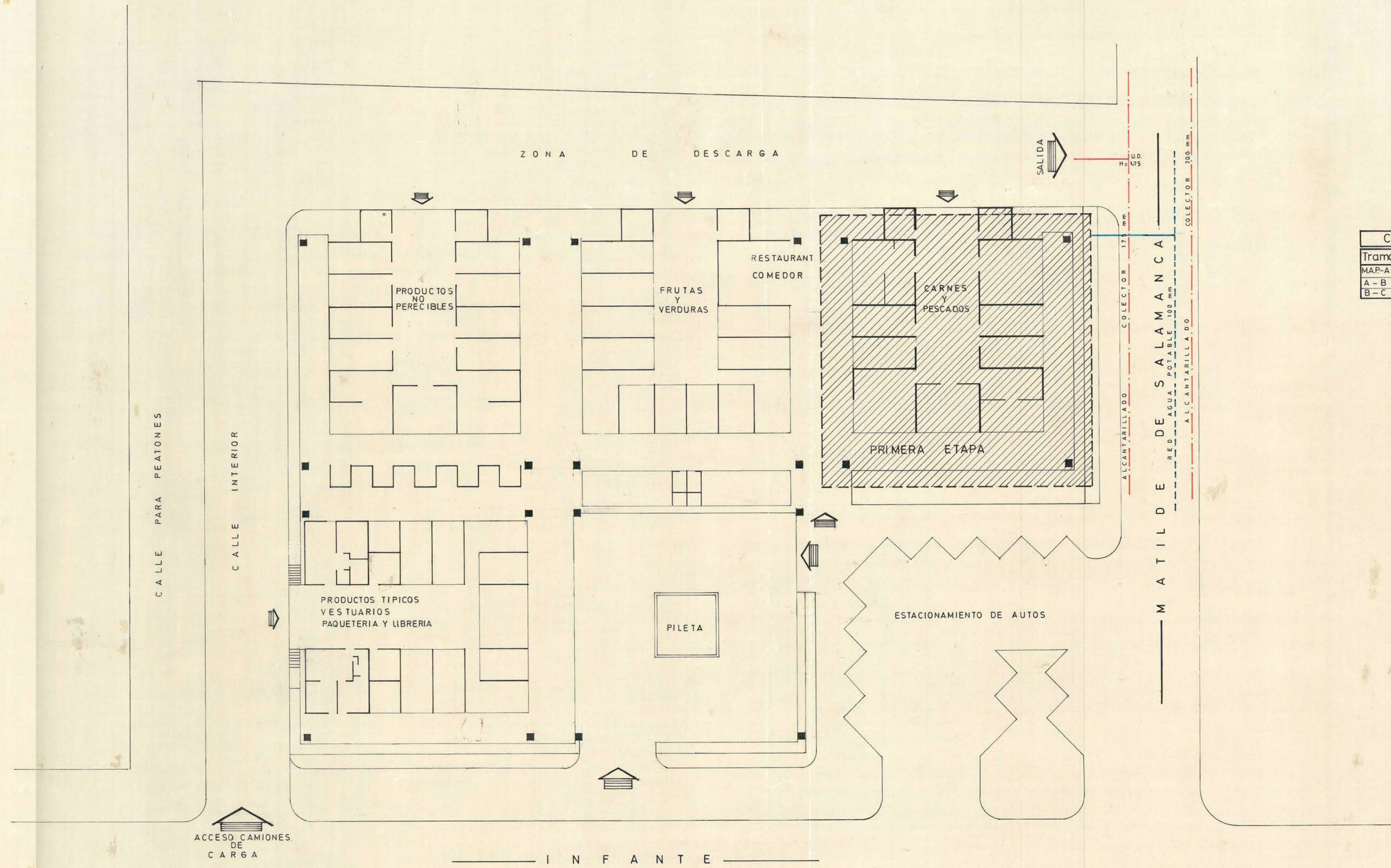
EMPLAZAMIENTO Escala 1:200
