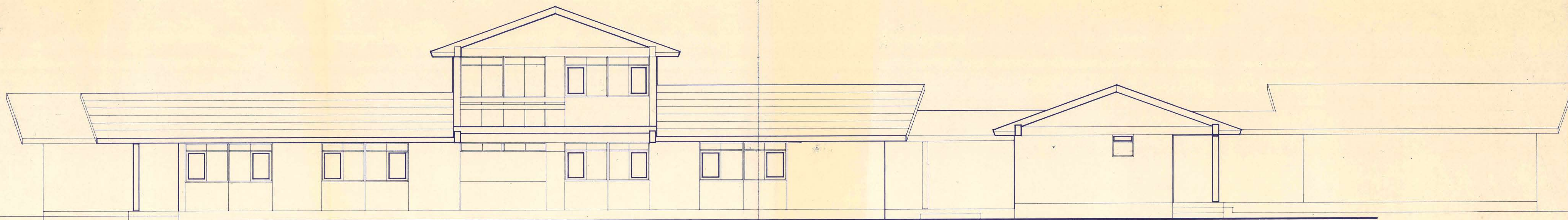
ELEVACION SUR
