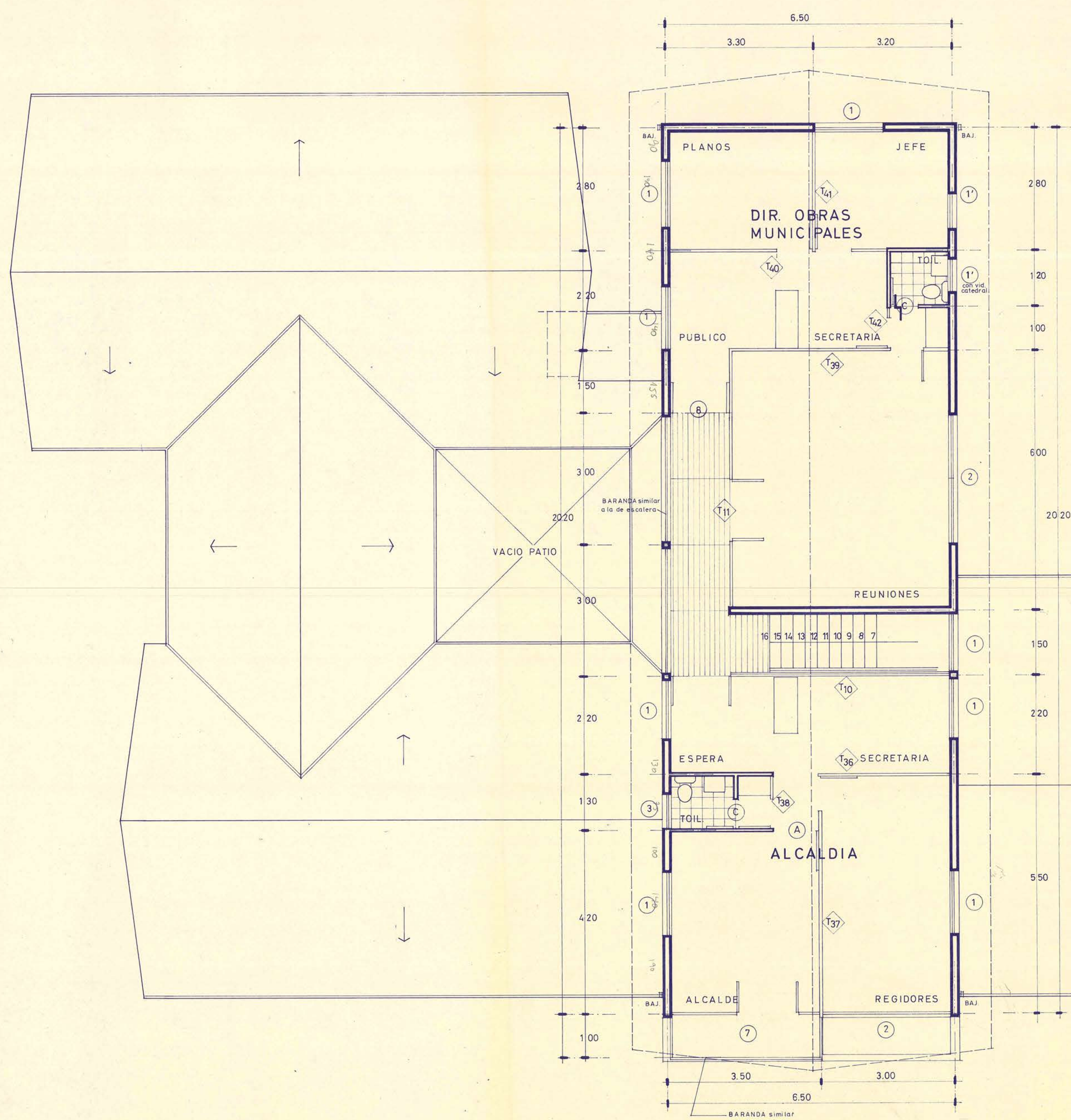
PLANTA SEGUNDO PISO
