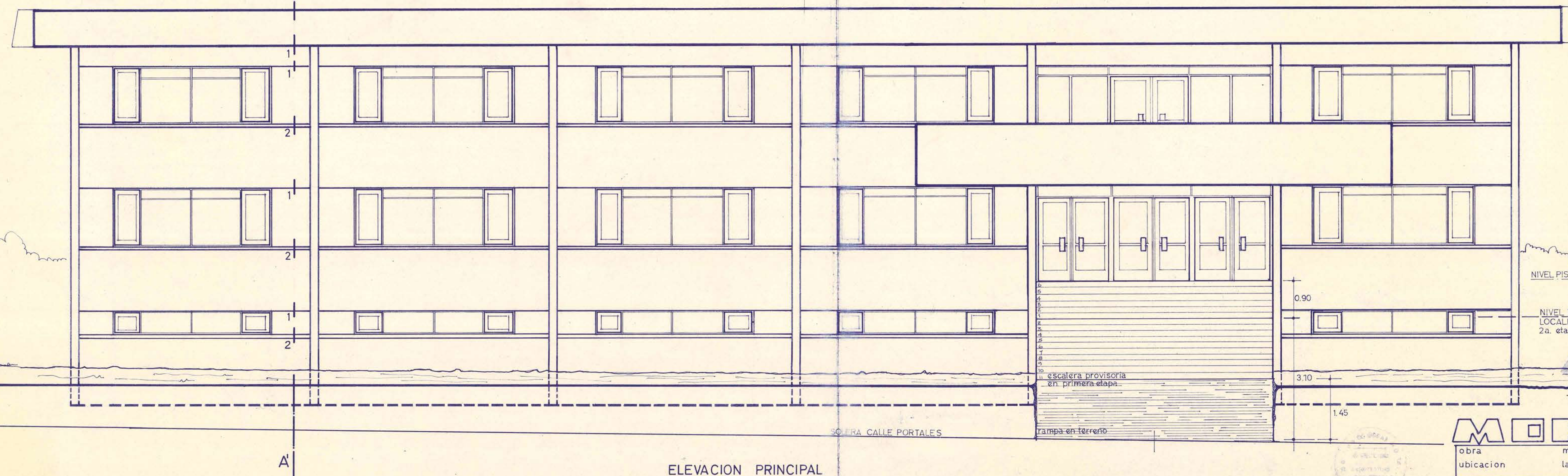
ELEVACION PRINCIPAL
