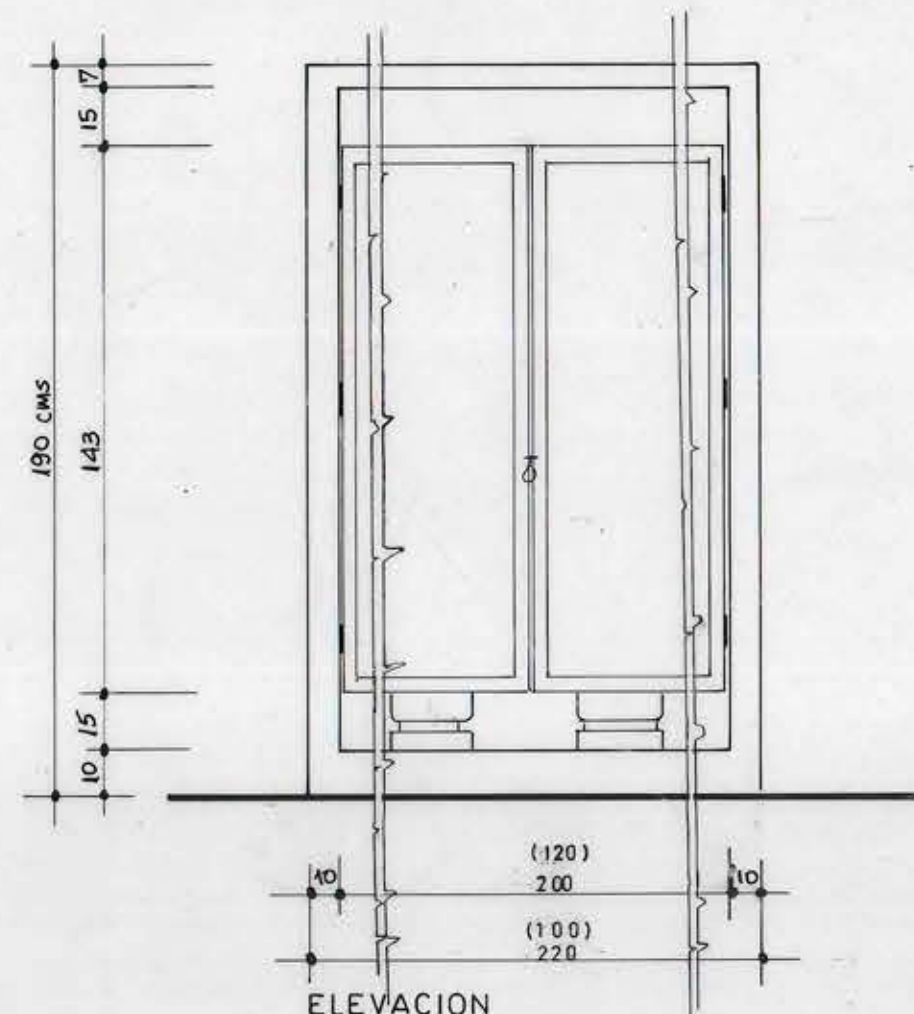
DETALLE CASETA DE GAS ESC. 1:20
