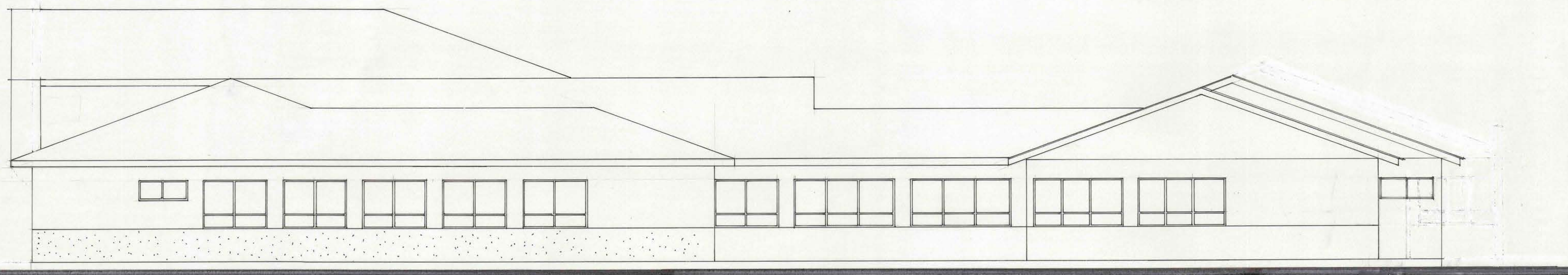
ELEV. ORIENTE ESC. 1:50
