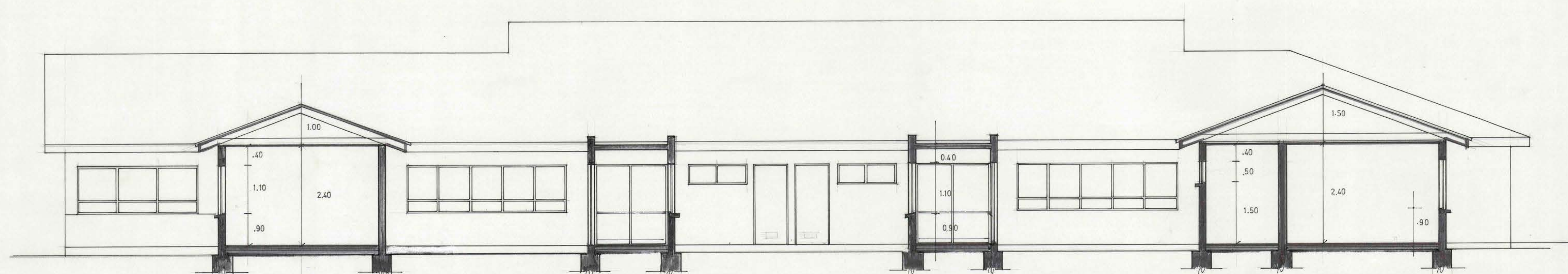
CORTE B-B ESC. 1:50
