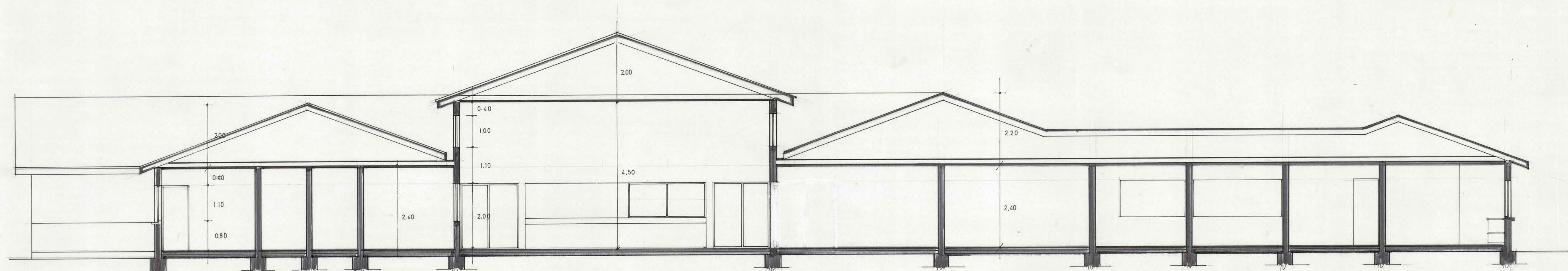
CORTE A-A ESC. 1:50
