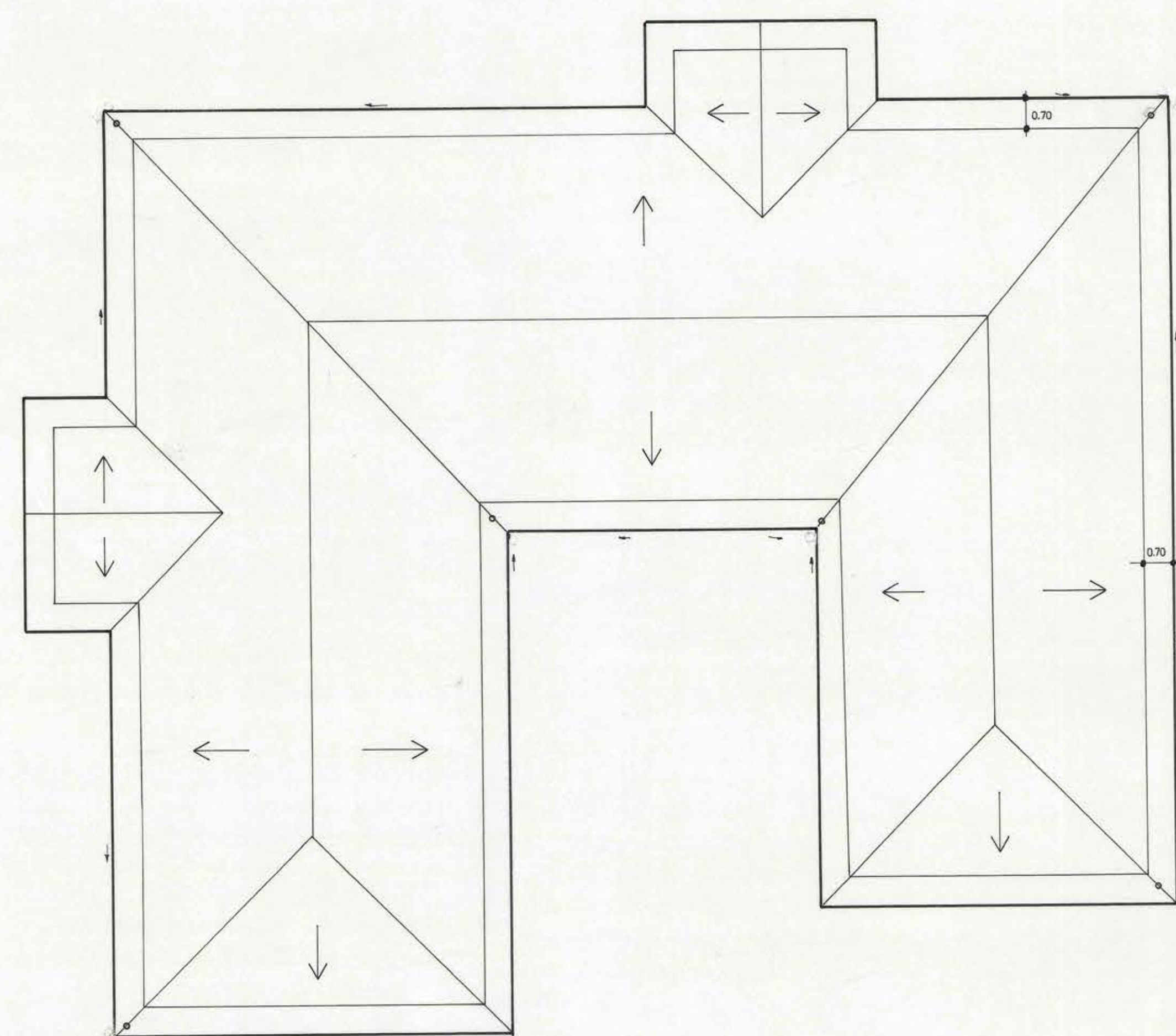
PLANTA DE TECHUMBRE ESCALA 1:100
