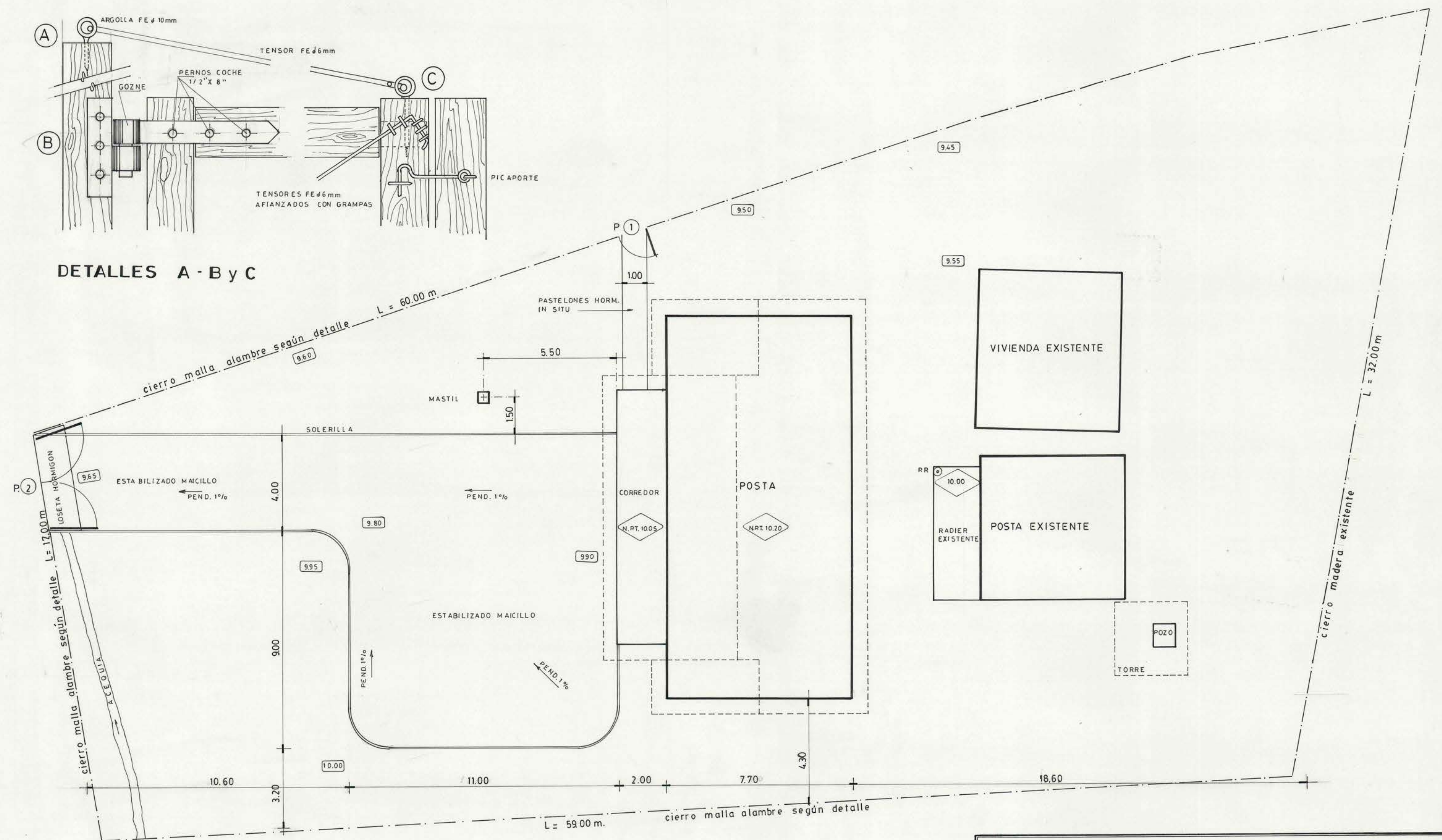
PLANTA DE : EMPLAZAMIENTO - NIVELES - PAVIMENTO Y - CIERROS ESC : 1:100
