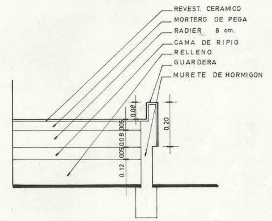
CORTE E. 1:10
