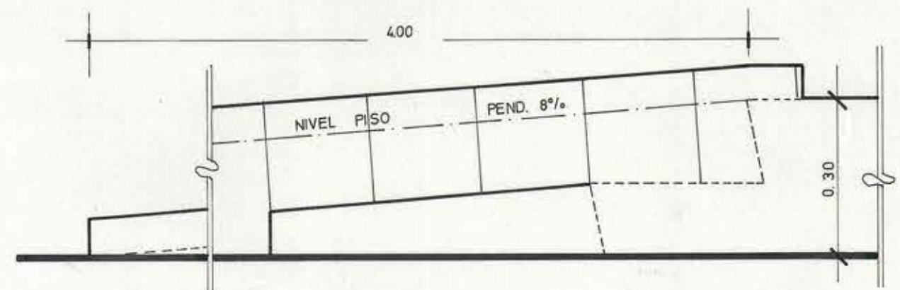
ELEVACION E. 1:10
