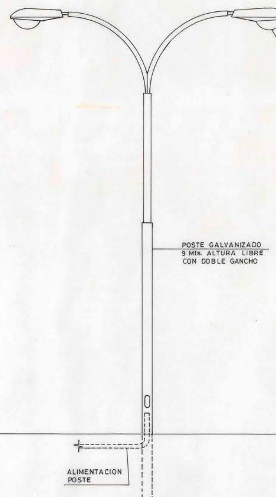
DETALLE POSTE CON LUMINARIA DOBLE
