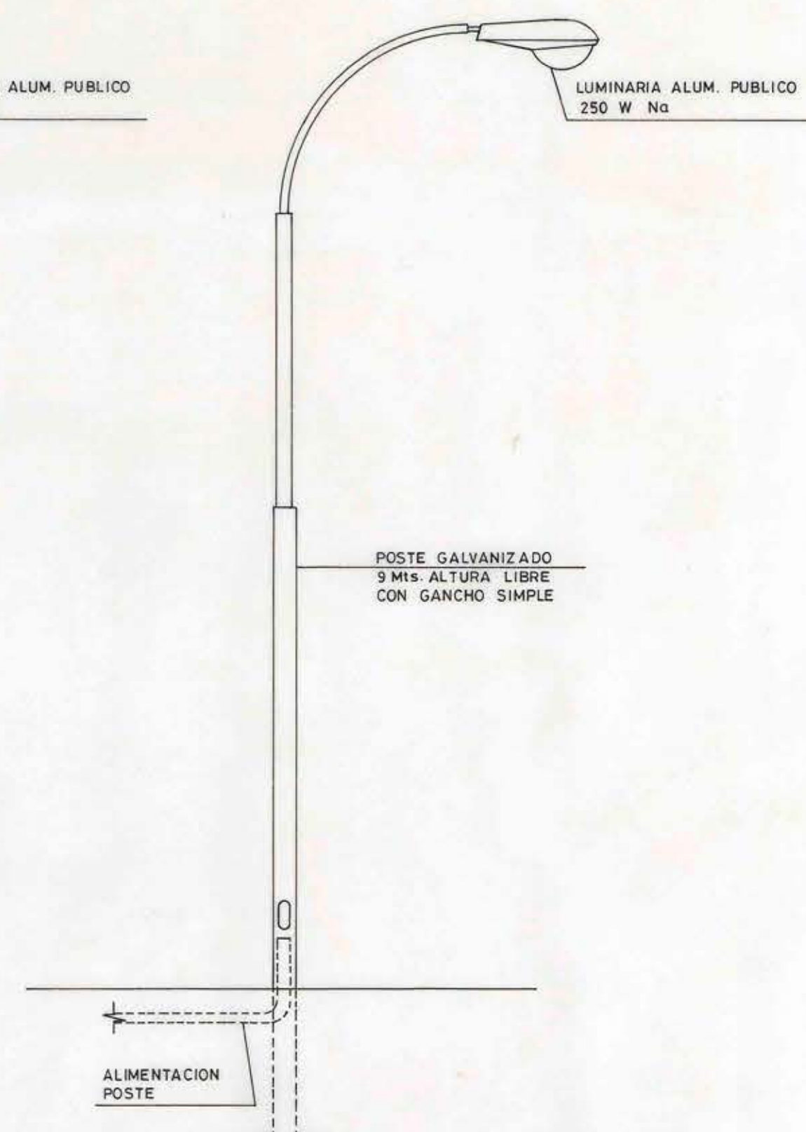
DETALLE POSTE CON LUMINARIA SIMPLE
