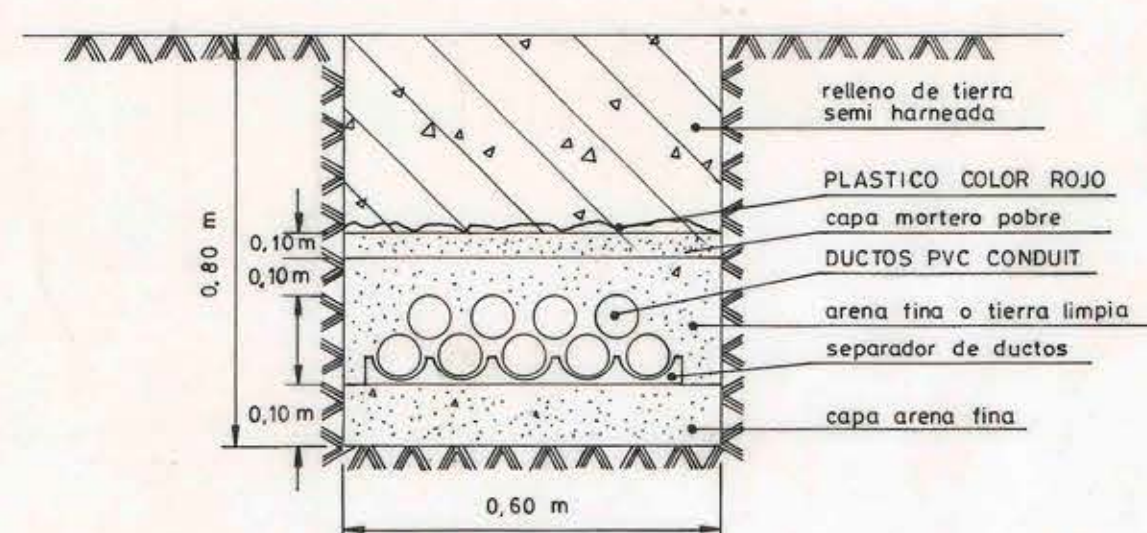
DETALLE ZANJA (TIPICO) (La cantidad de ductos es solo esquemática)
