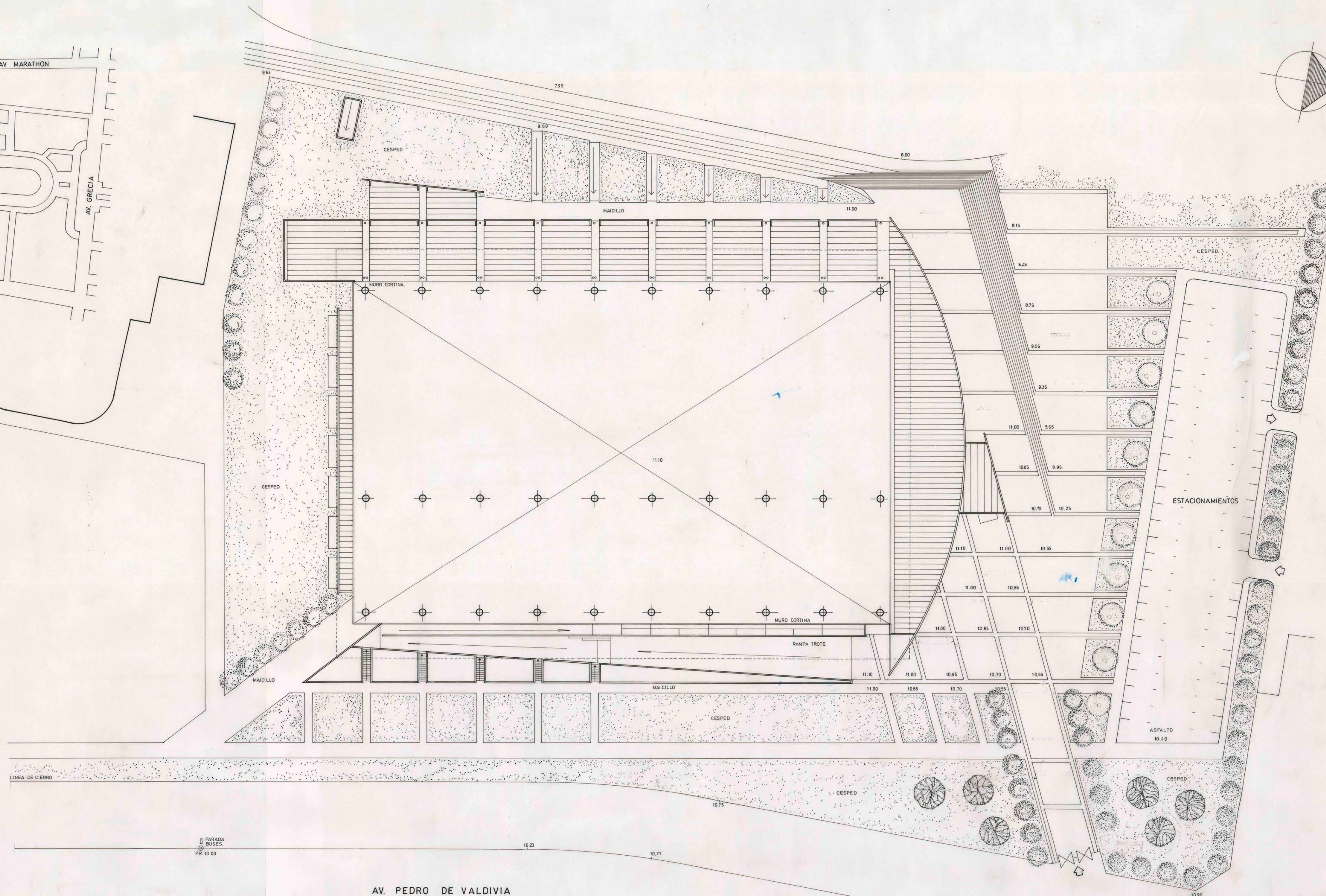
EMPLAZAMIENTO ESCALA 1:250
