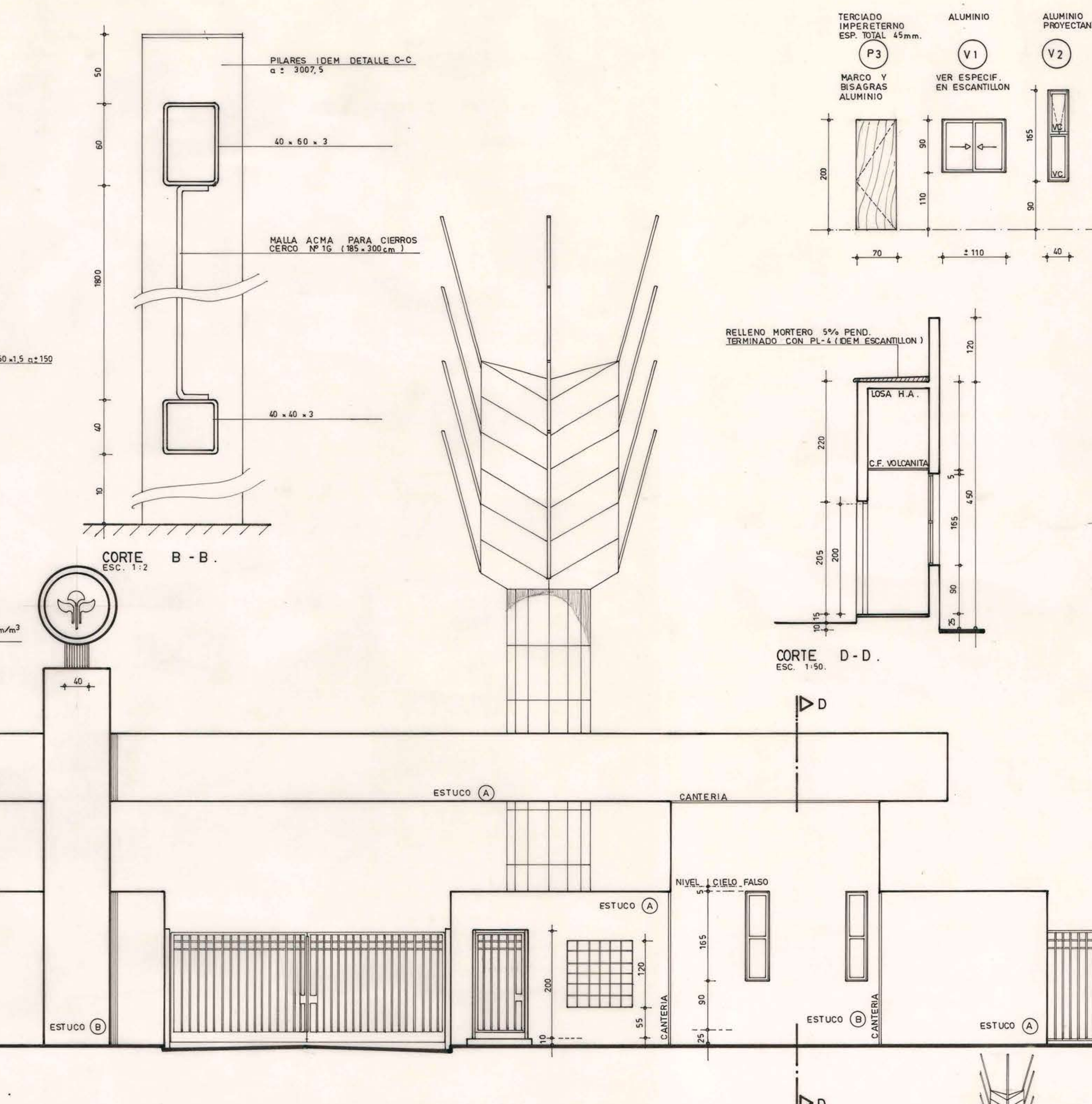
ELEVACION CIERRO A LA CARRETERA ESC. 1:200
