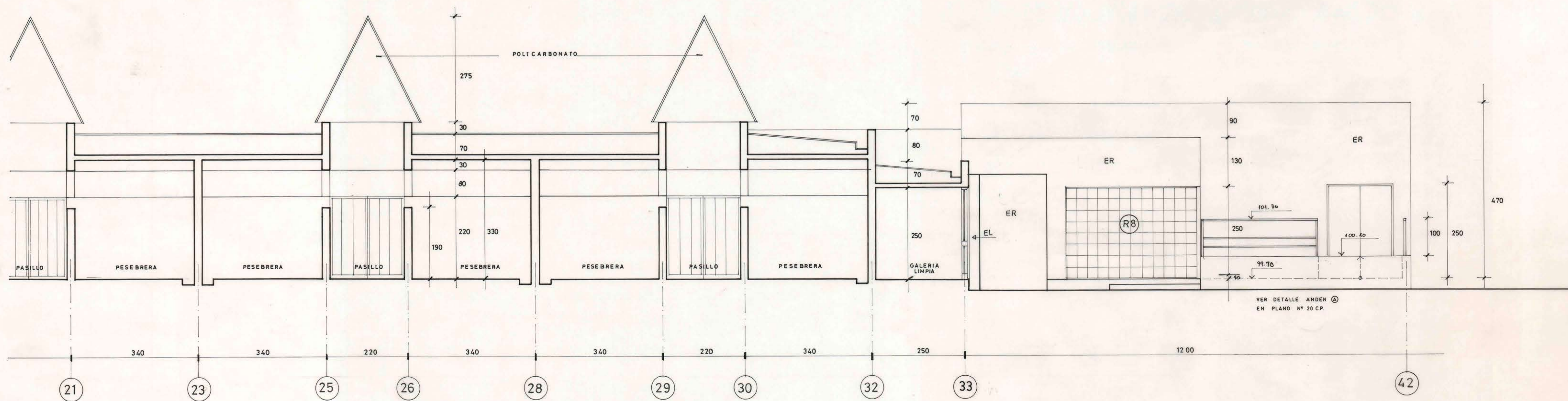
CORTE B-B
