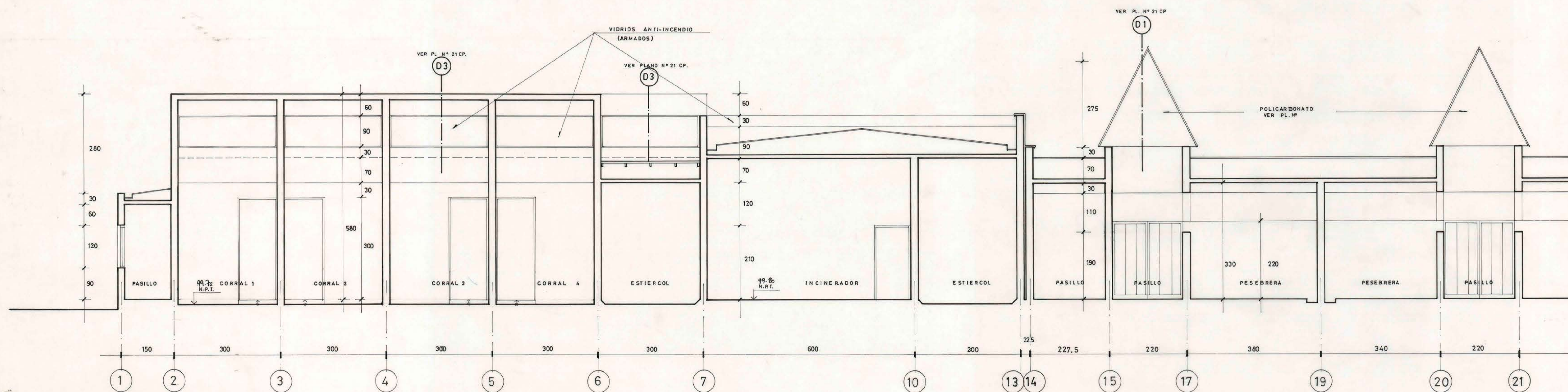
CORTE B-B
