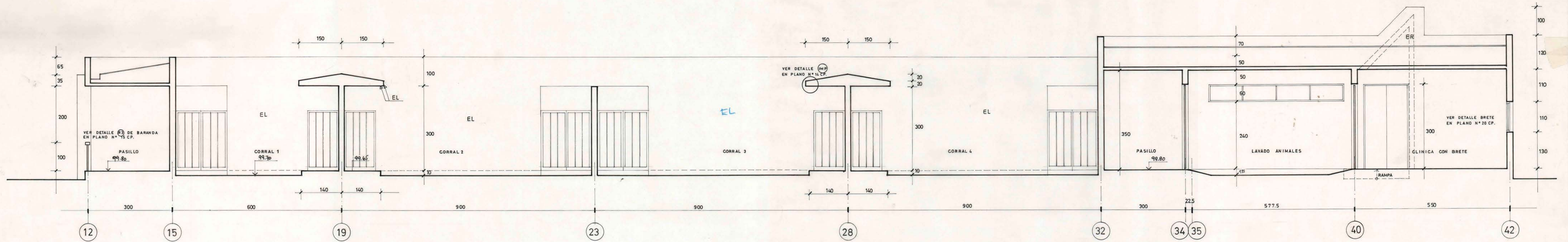
CORTE A-A
