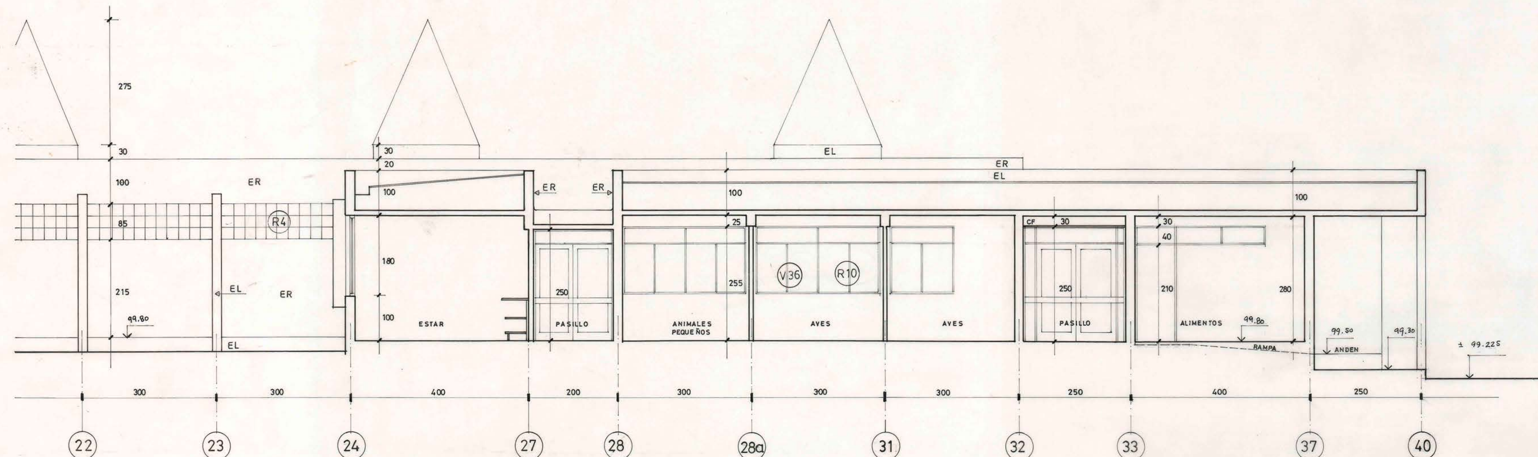
CORTE - ELEVACION C-C
