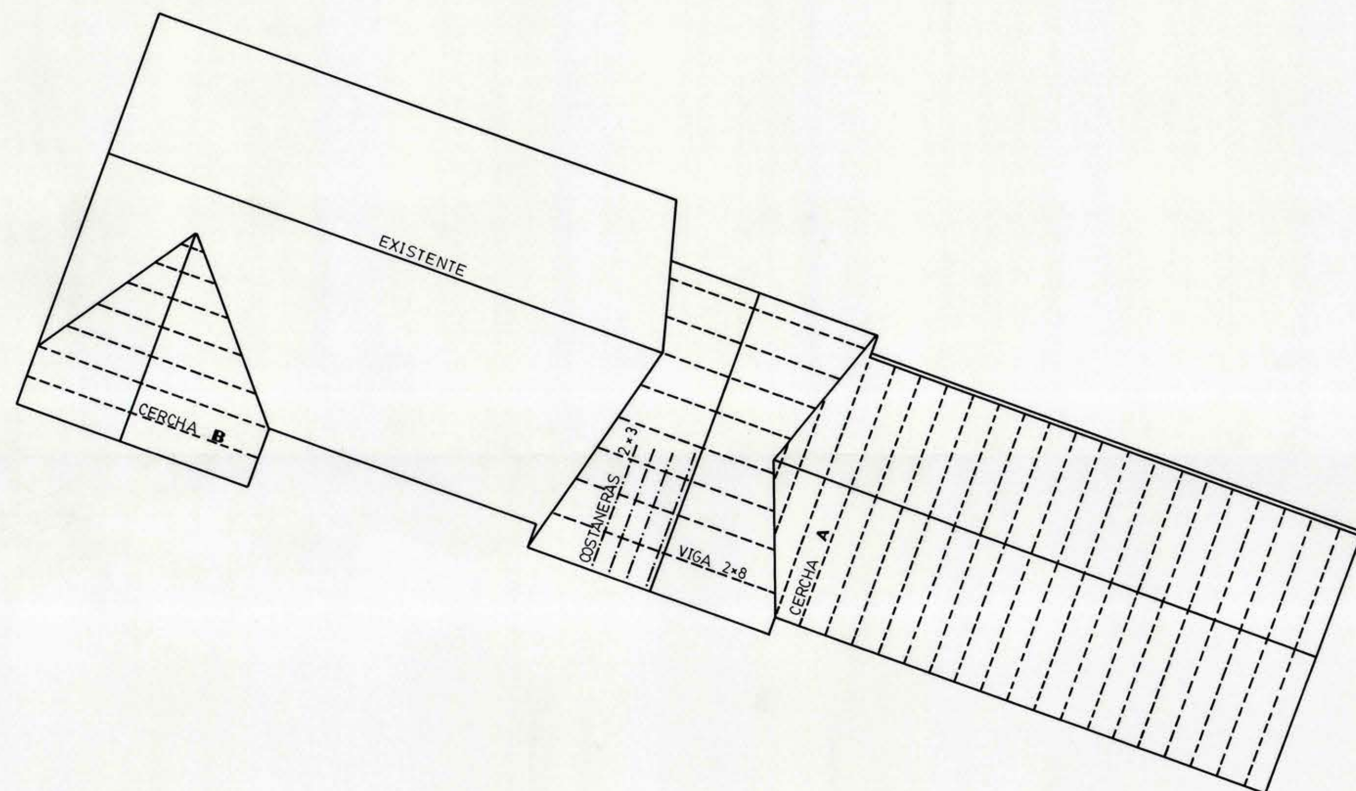
TECHUMBRE Esc. 1/100
