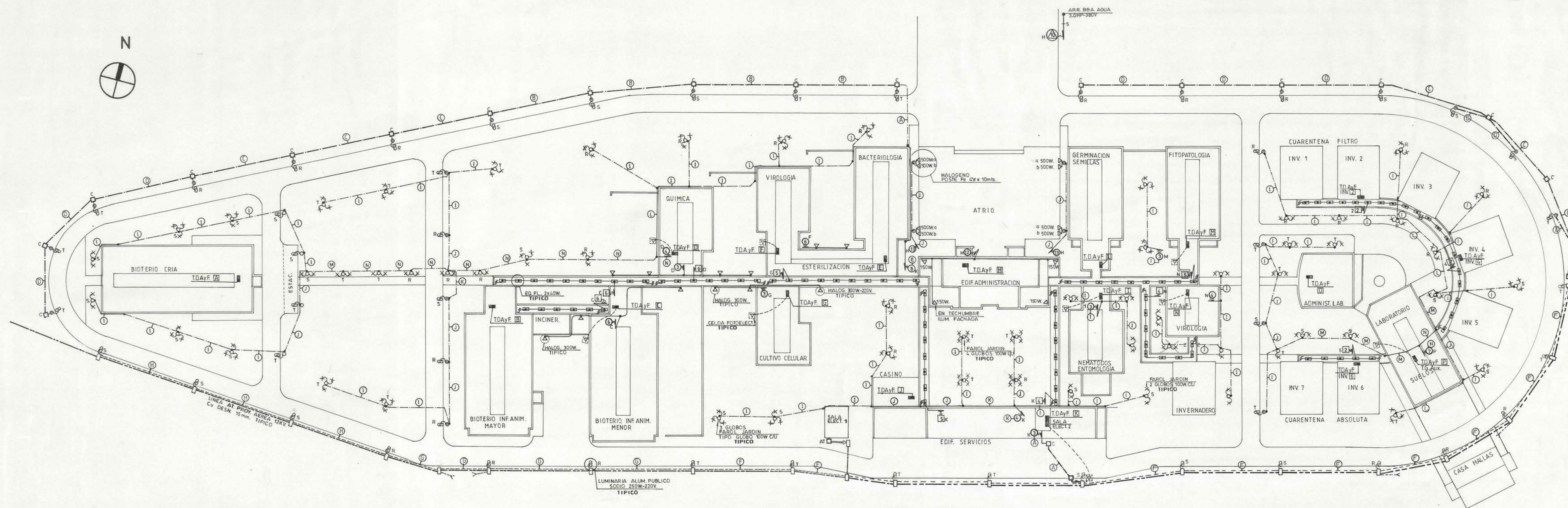
PLANTA GENERAL (Alumbrado Exterior) ESCALA: 1:500
