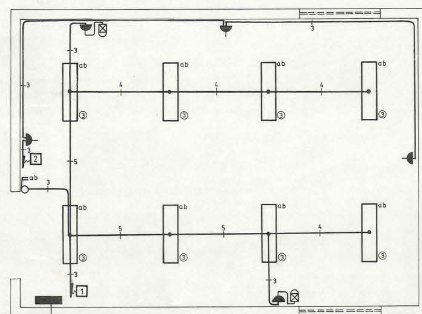
SALA ELECTRICA 1 ESCALA: 1:50
