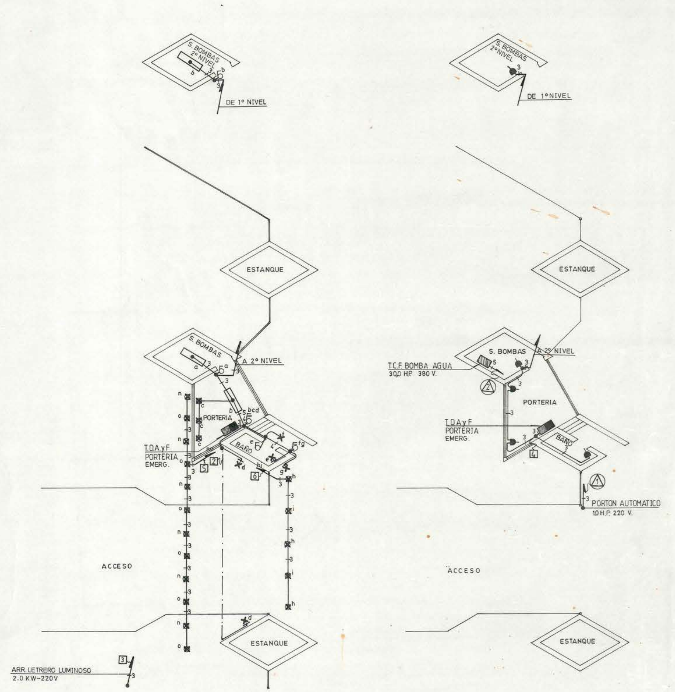
PLANTA PORTERIA (ALUMBRADO) ESCALA: 1:100
