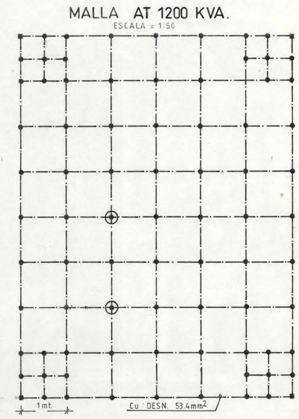
MALLA AT 150 y 250 KVA. ESCALA: 1:50
