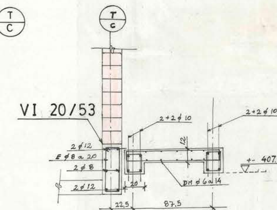
SECCION 1-1
