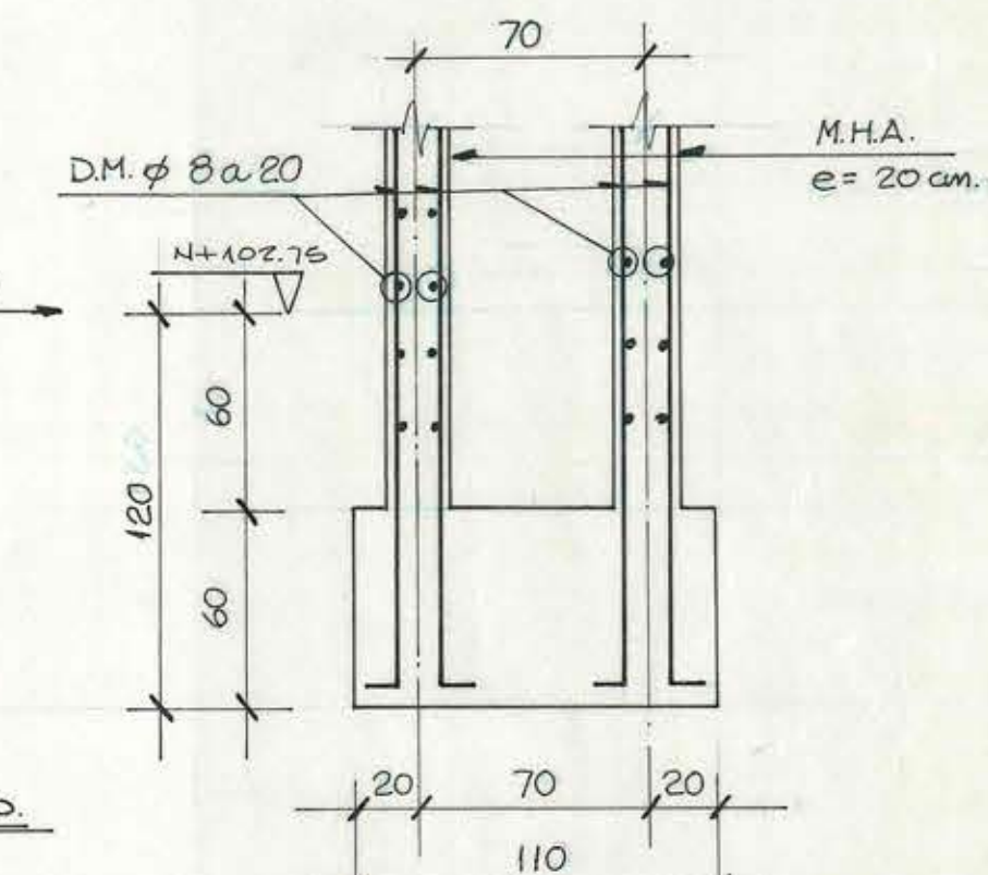
SECCION A-A
