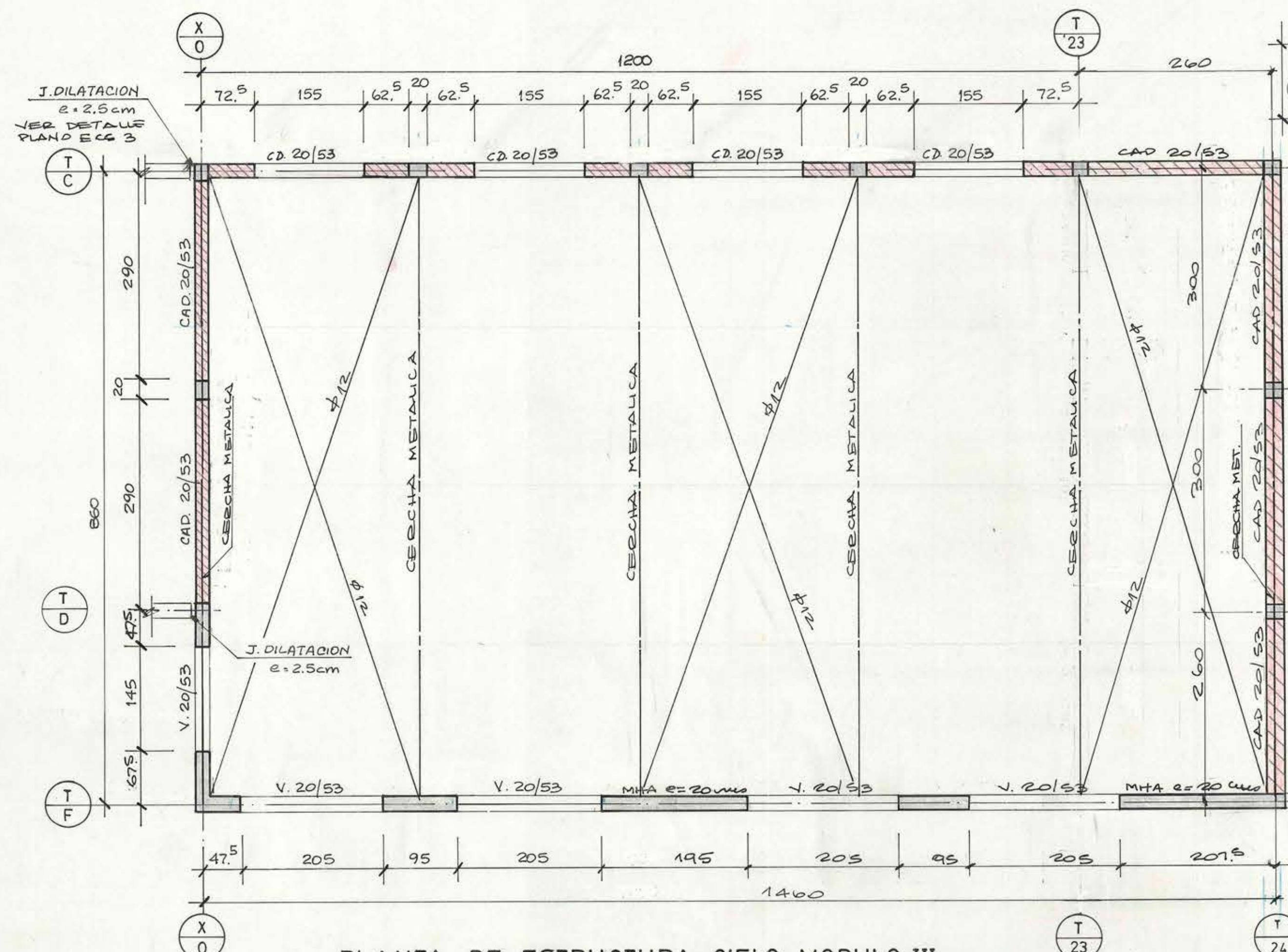
PLANTA DE ESTRUCTURA CIELO MODULO III
