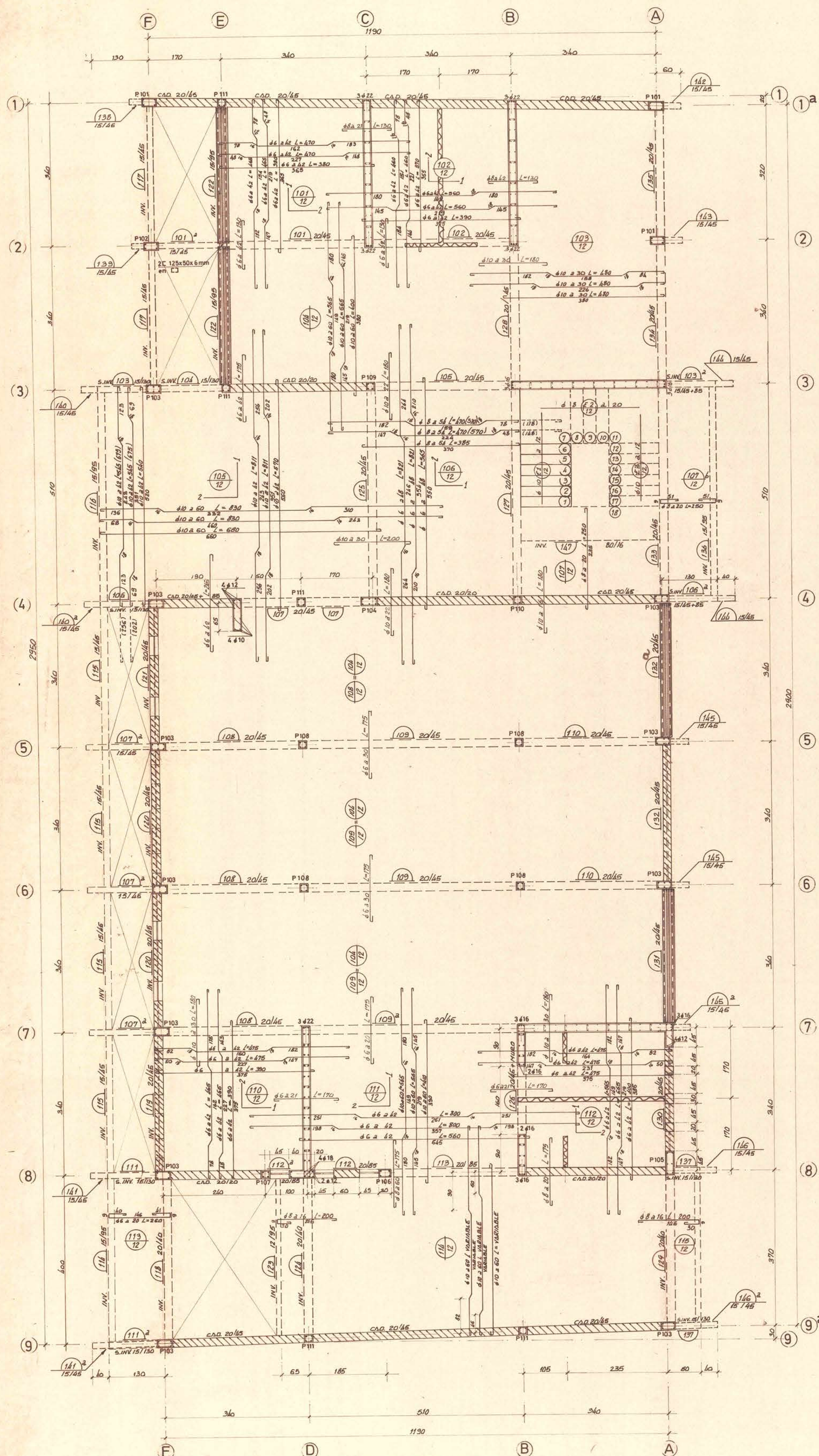
PLANTA DE ESTRUCTURA Y LOSAS CIELO DEL 1er. PISO. NOTA: Reparticiones en Losas \phi 6 a 25
