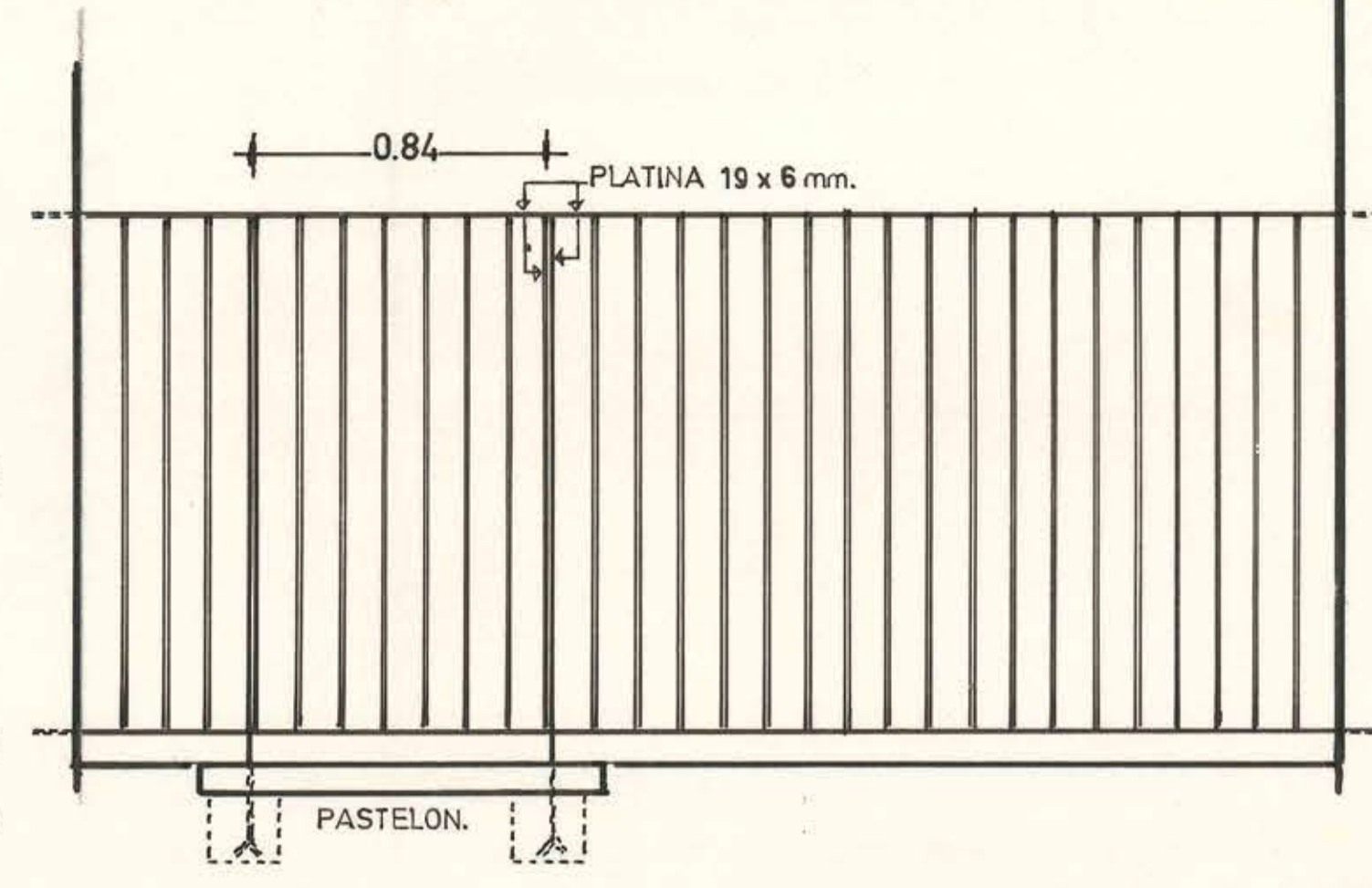
DETALLE DE REJA DE CIERRE ESC. 1:20
