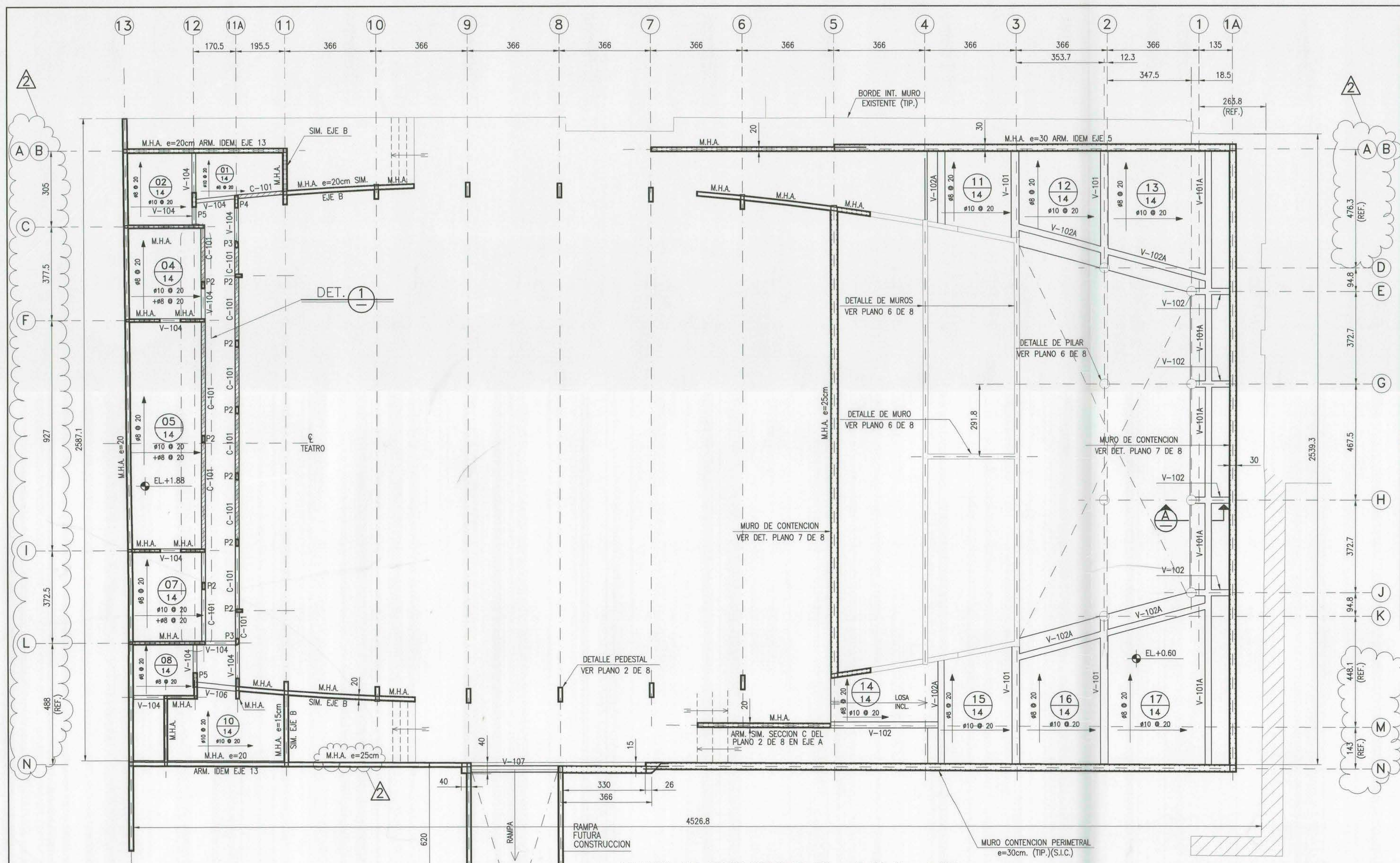
PLANTA DE ESTRUCTURAS EL. +0.60 Y +1.88 ESCALA 1:75
