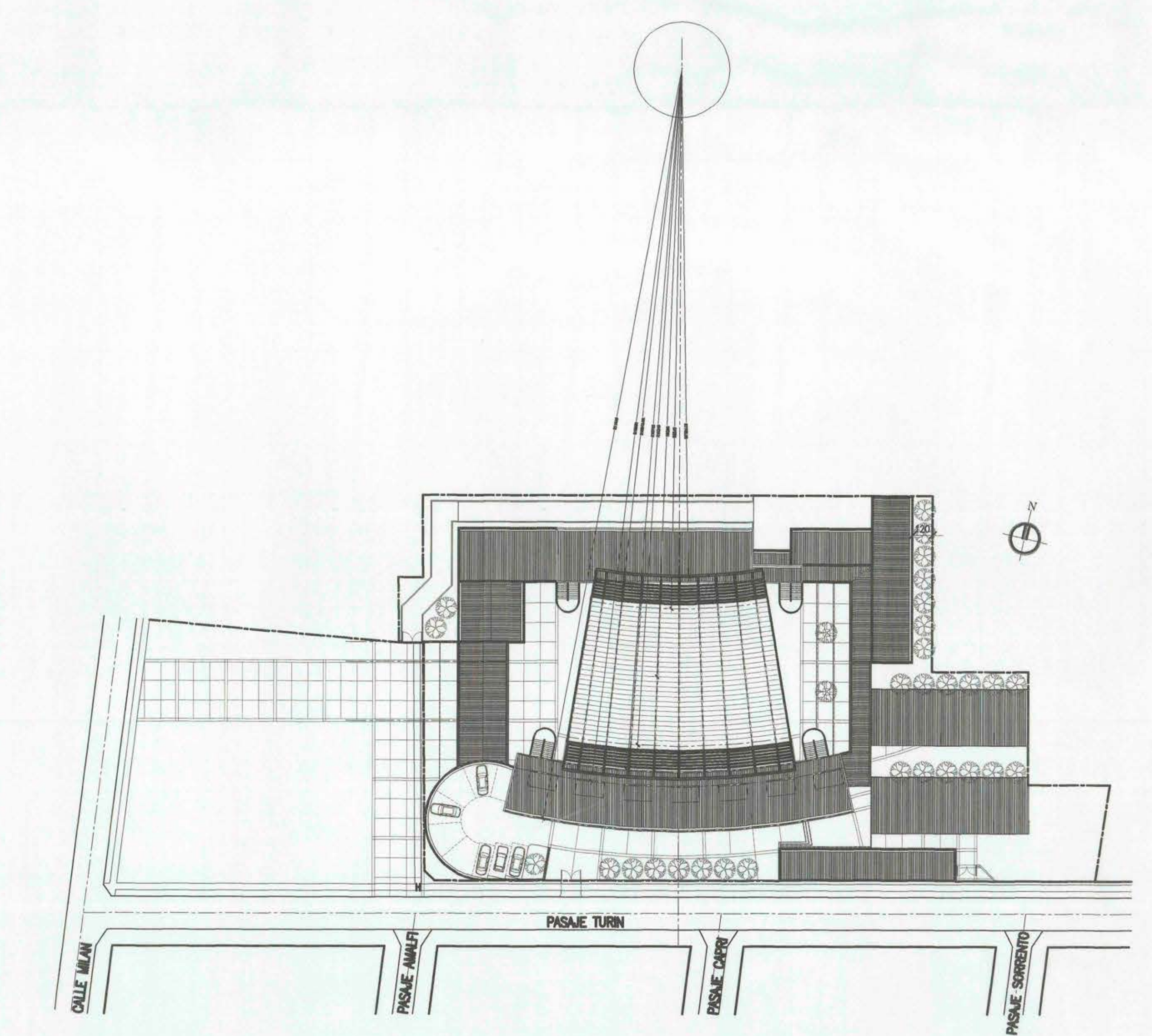
PLANTA GENERAL DE UBICACION ESC. 1/500
