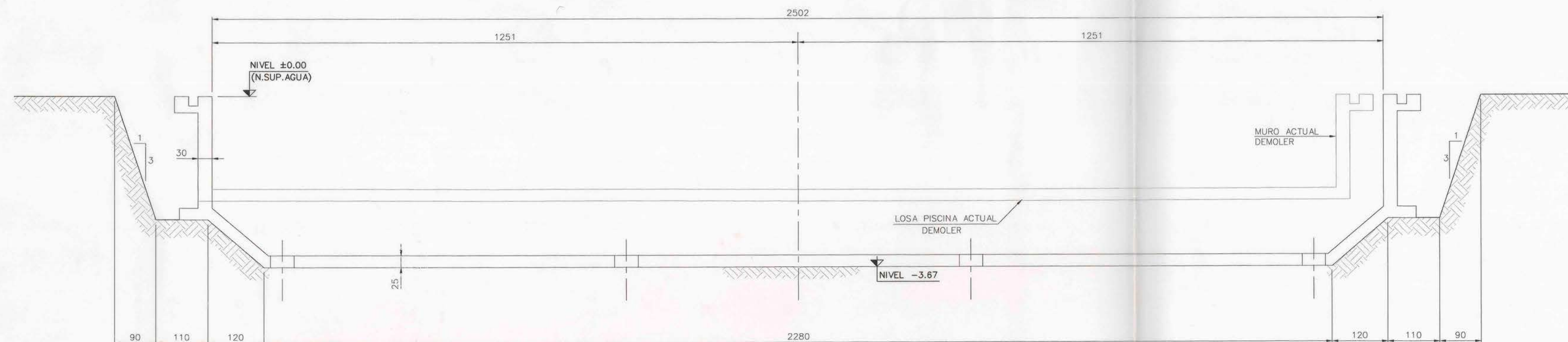
SECCION TRANSVERSAL PISCINA NORTE-EXCAVACIONES ESCALA 1:100
