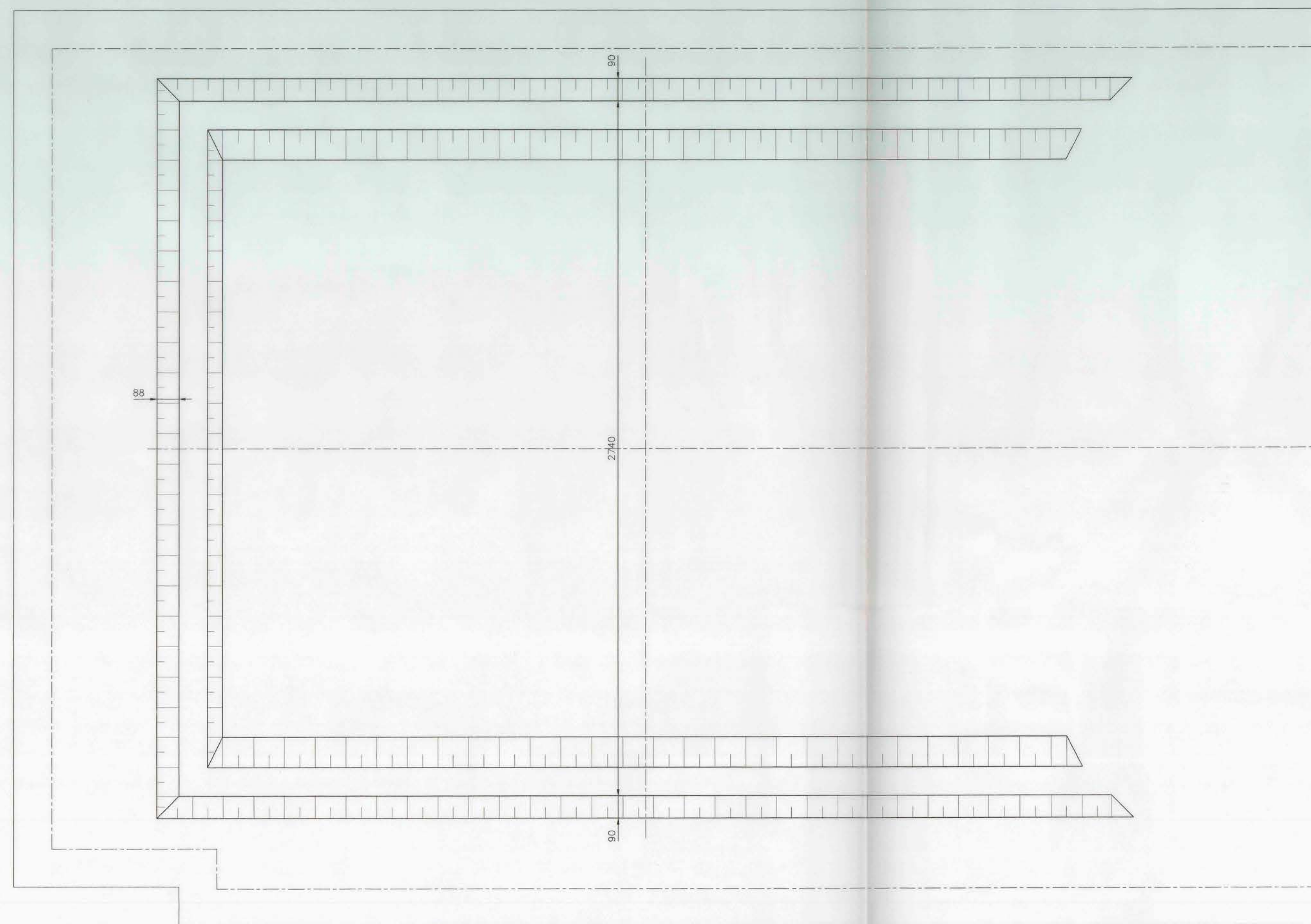
PLANTA DE EXCAVACIONES PISCINA NORTE ESCALA 1:100
