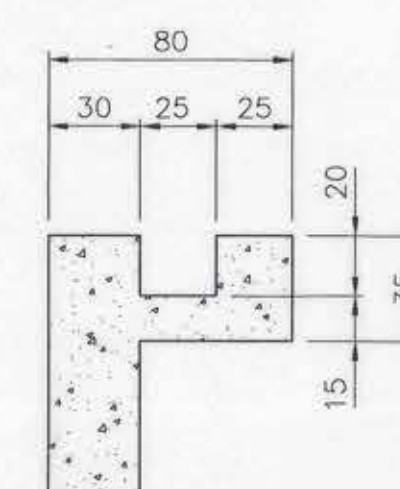
DETALLE 1 ESCALA 1:25
