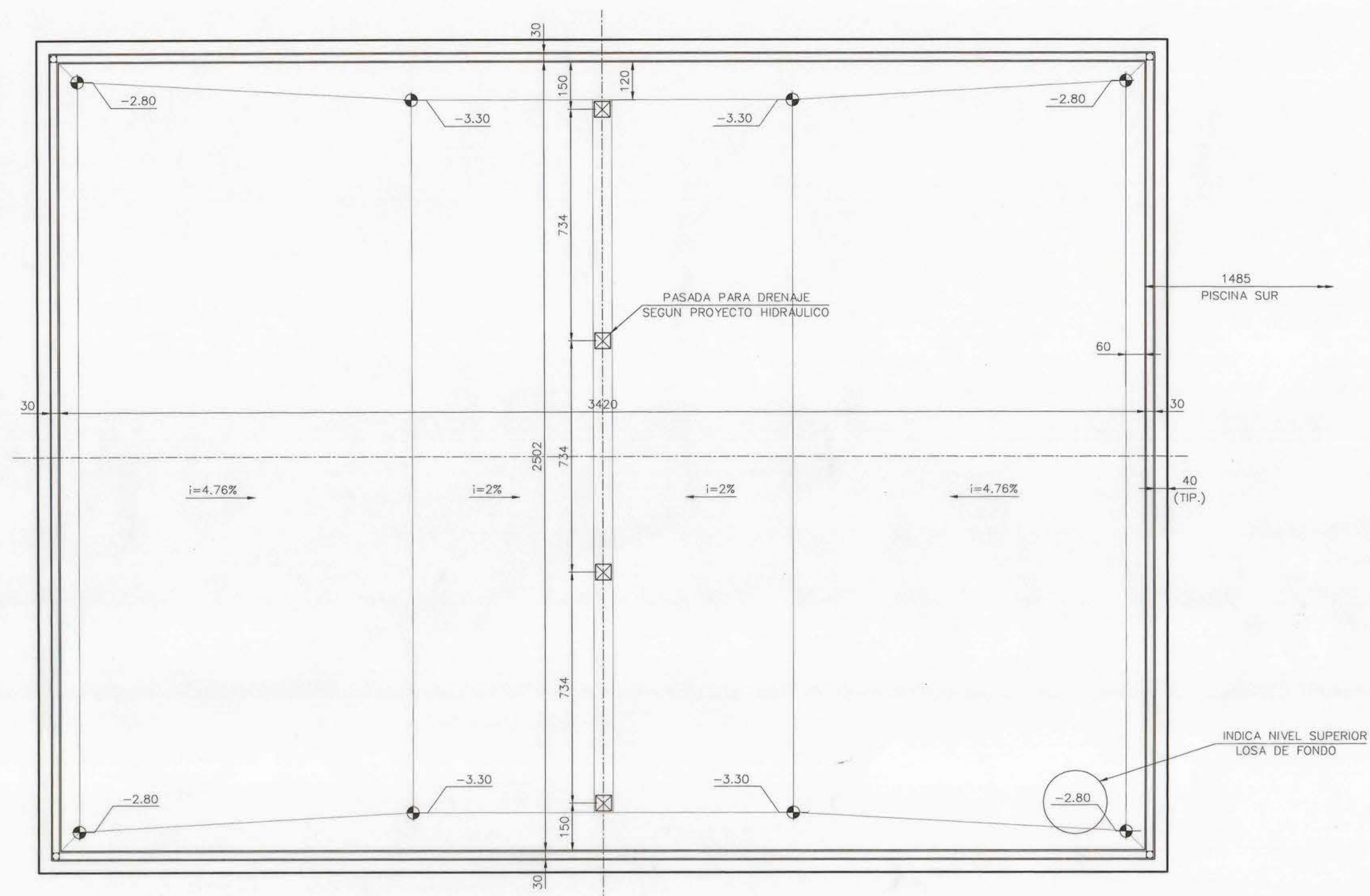
PLANTA DE FUNDACIONES PISCINA NORTE ESCALA 1:100
