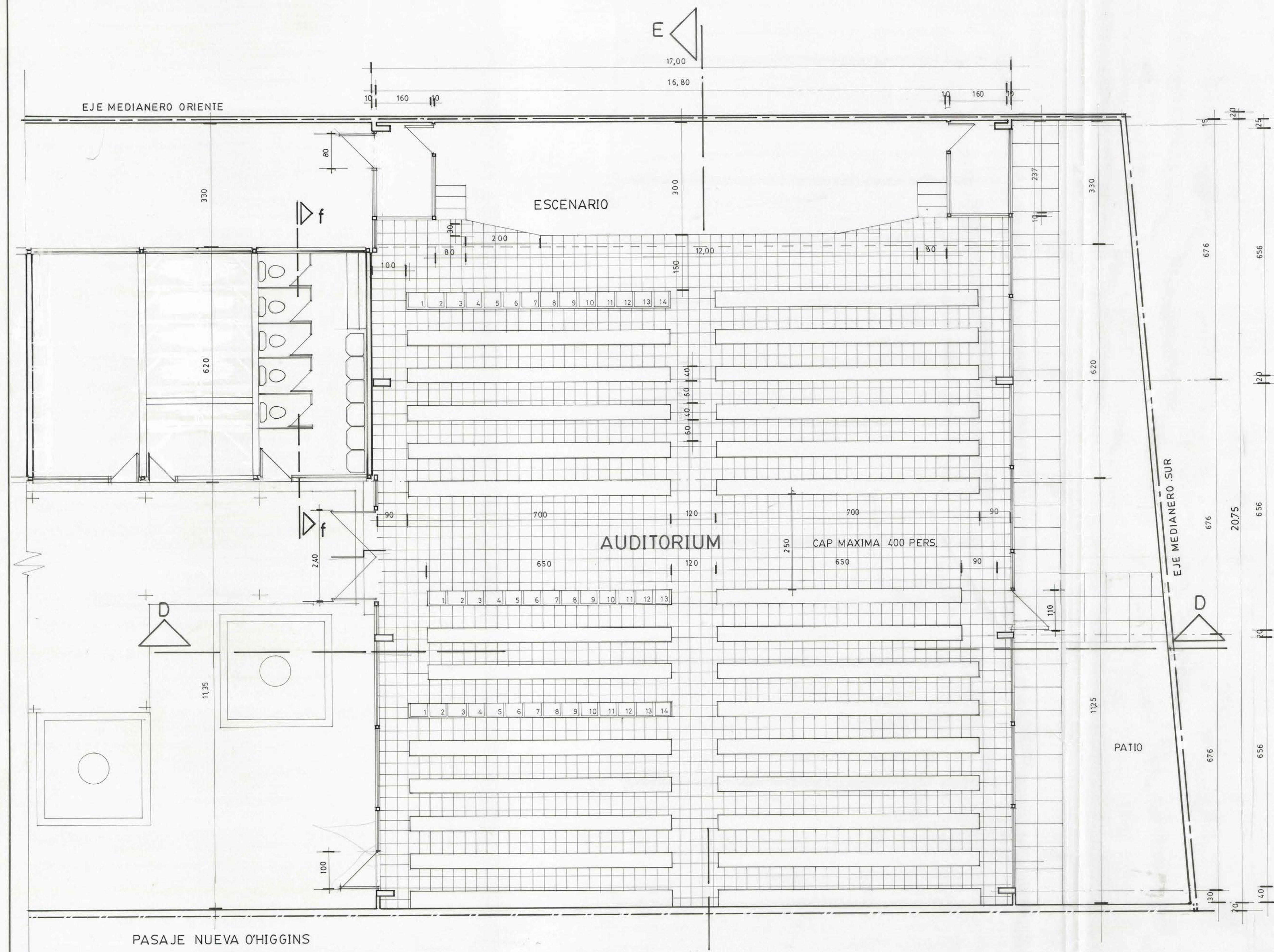
PLANTA AUDITORIUM
