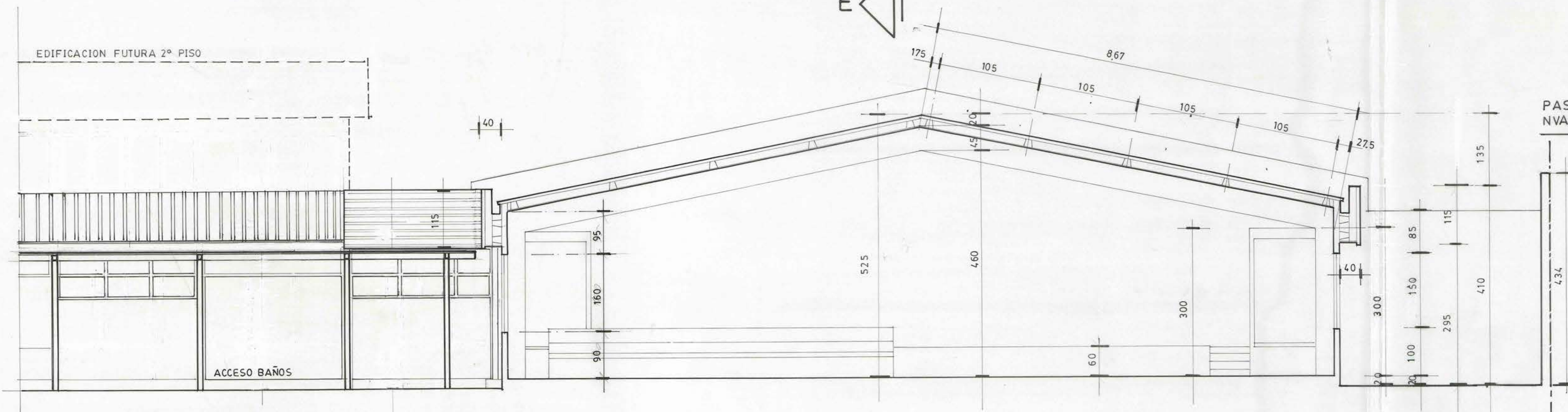
CORTE D-D
