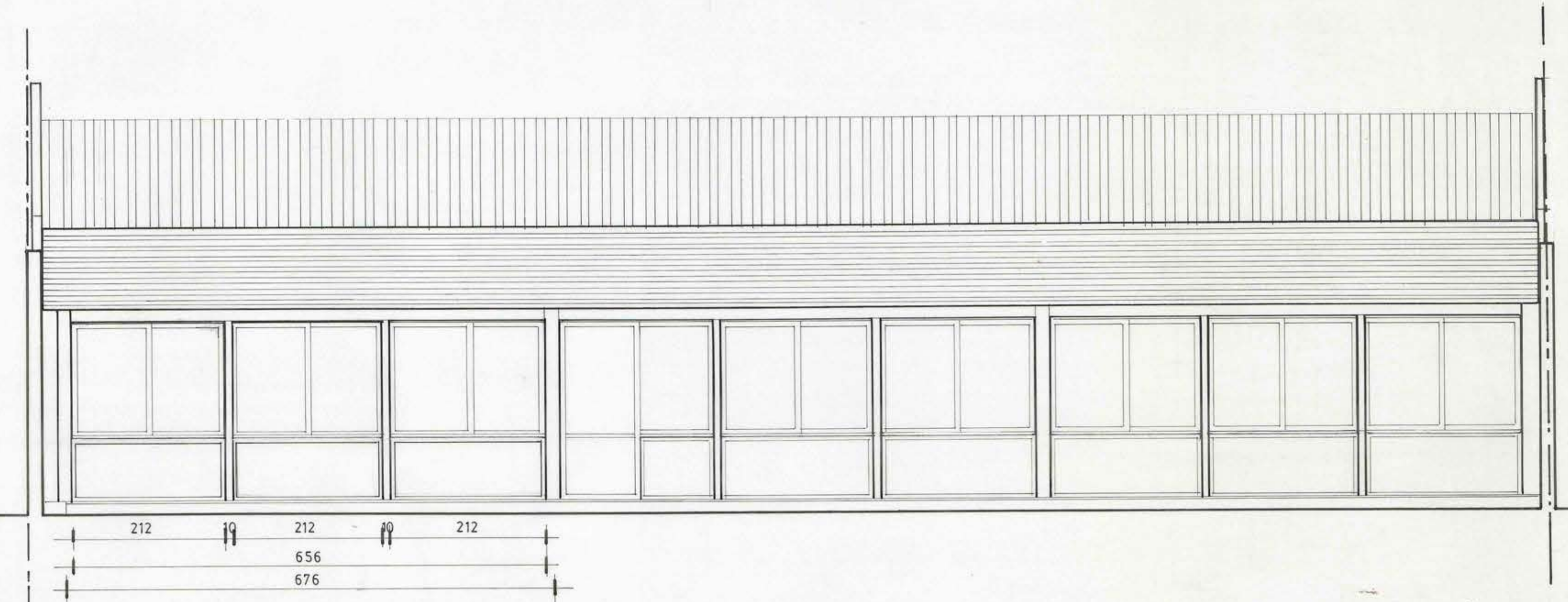
ELEVACION SUR
