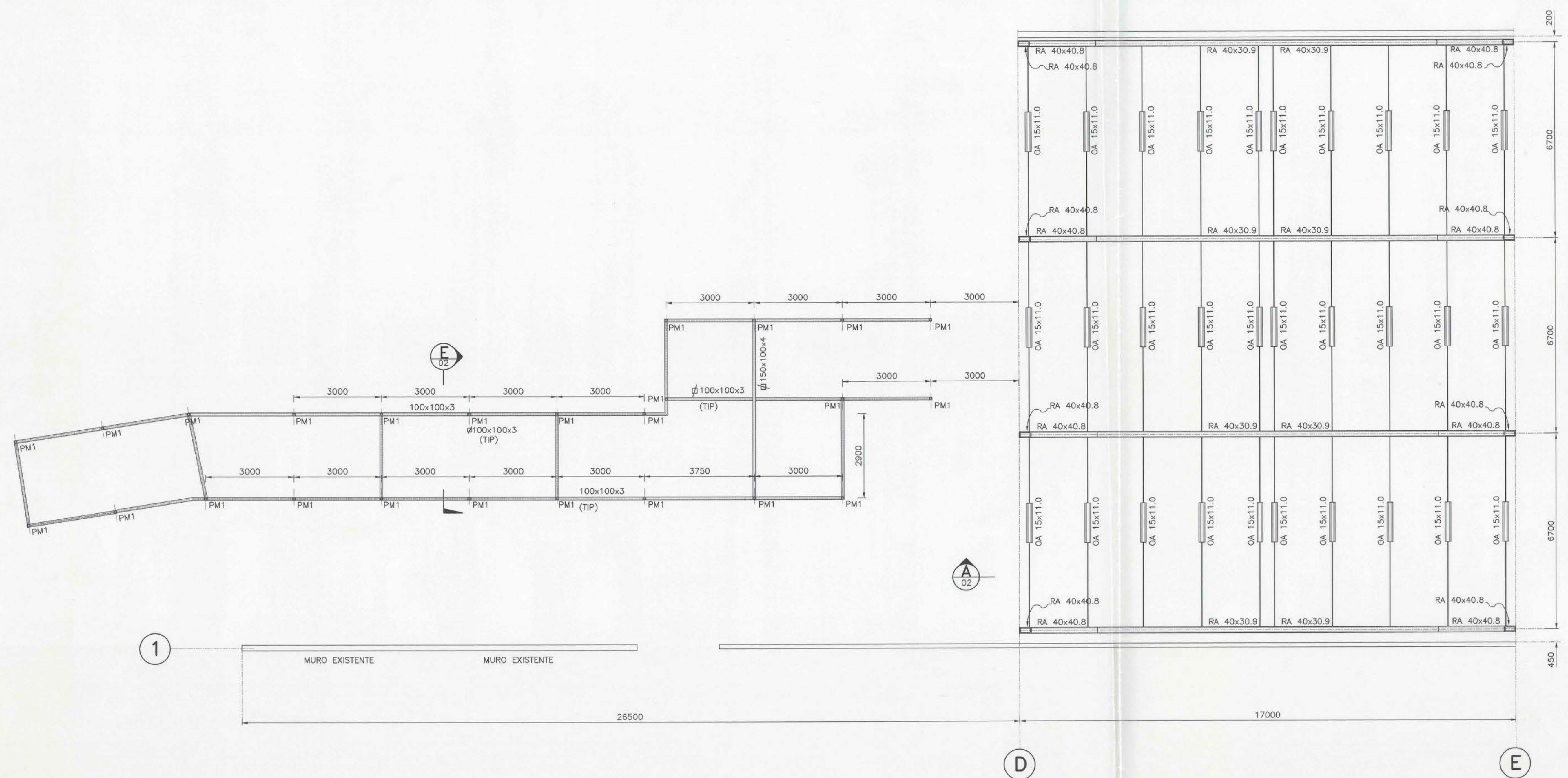
PLANTA DE ESTRUCTURAS ESC. 1:75
