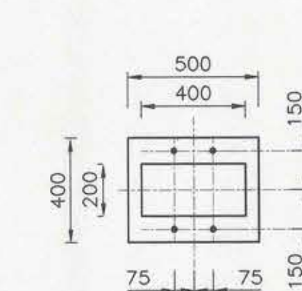
SECCION B ESC. 1:20
