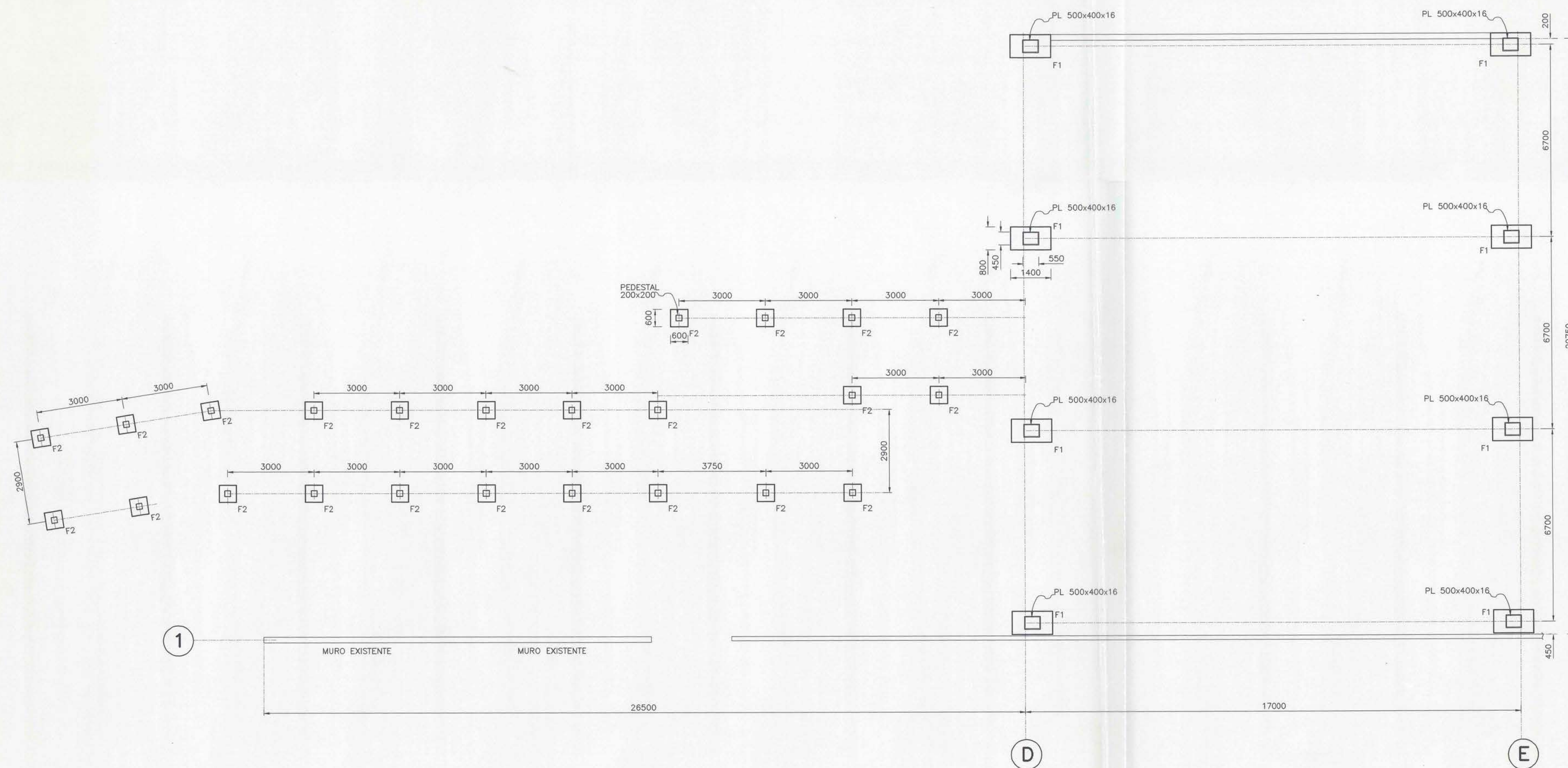
PLANTA DE FUNDACIONES ESC. 1:75
