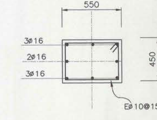
SECCION C ESC. 1:20
