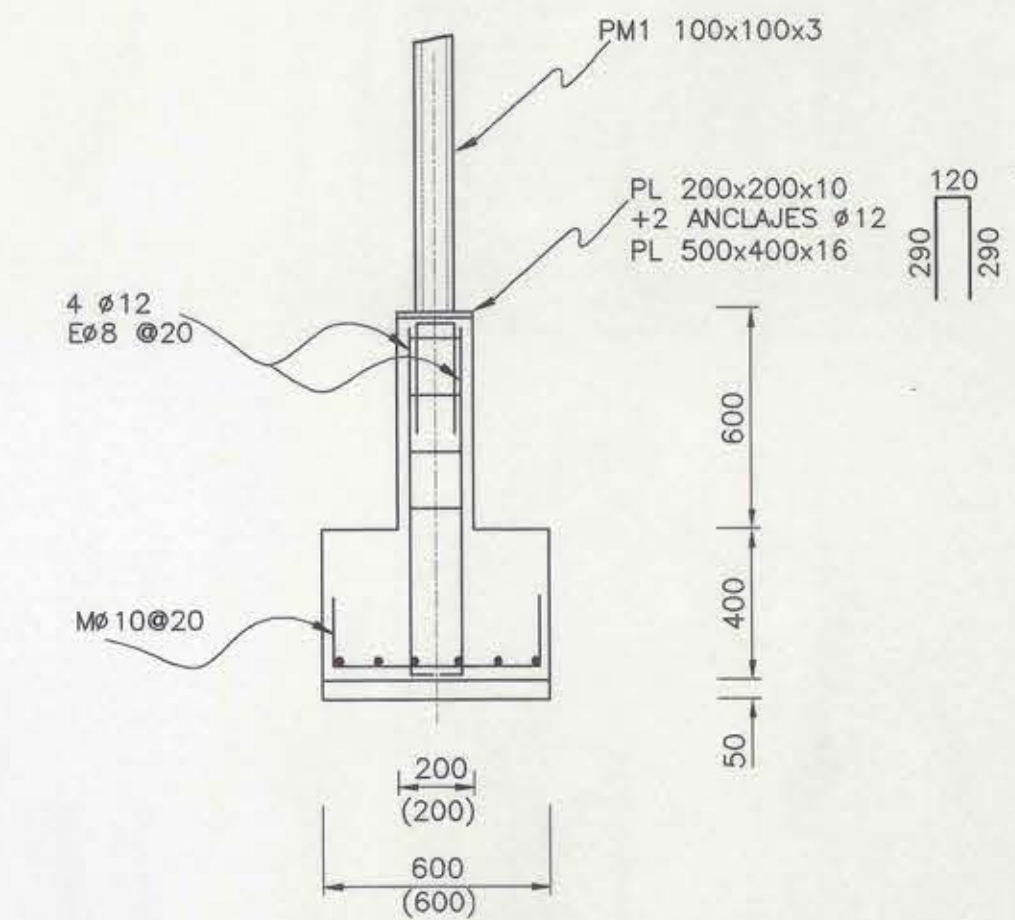
DETALLE FUNDACION F2 ESC. 1:20
