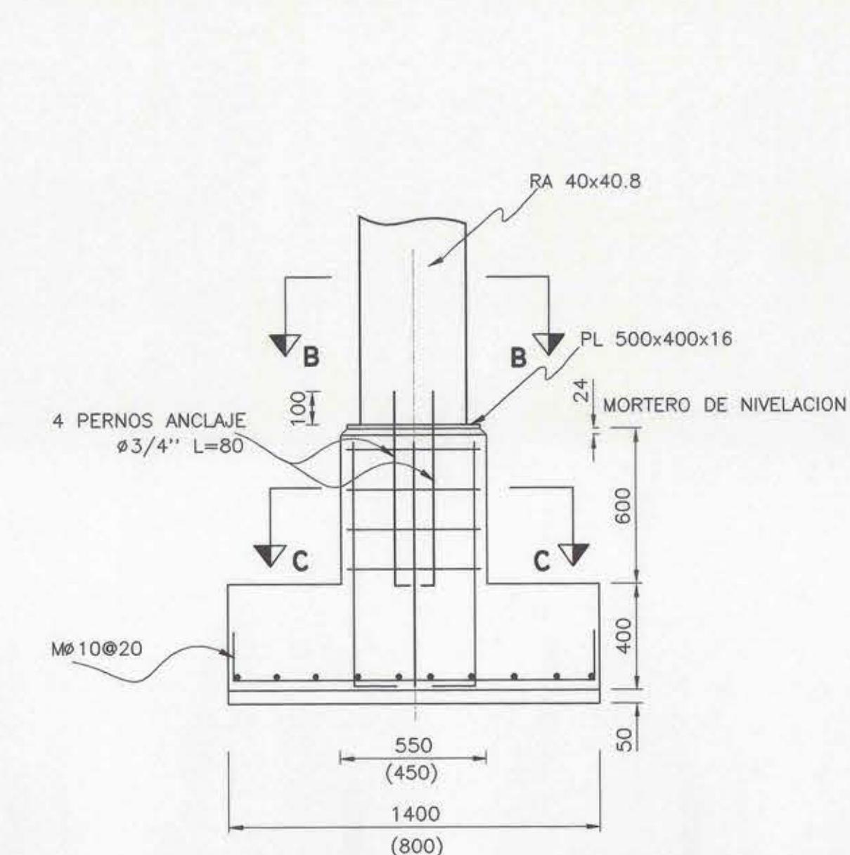
DETALLE FUNDACION F1 ESC. 1:20
