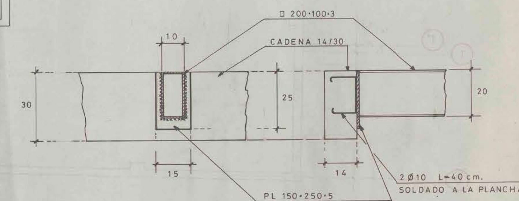
DET. B
