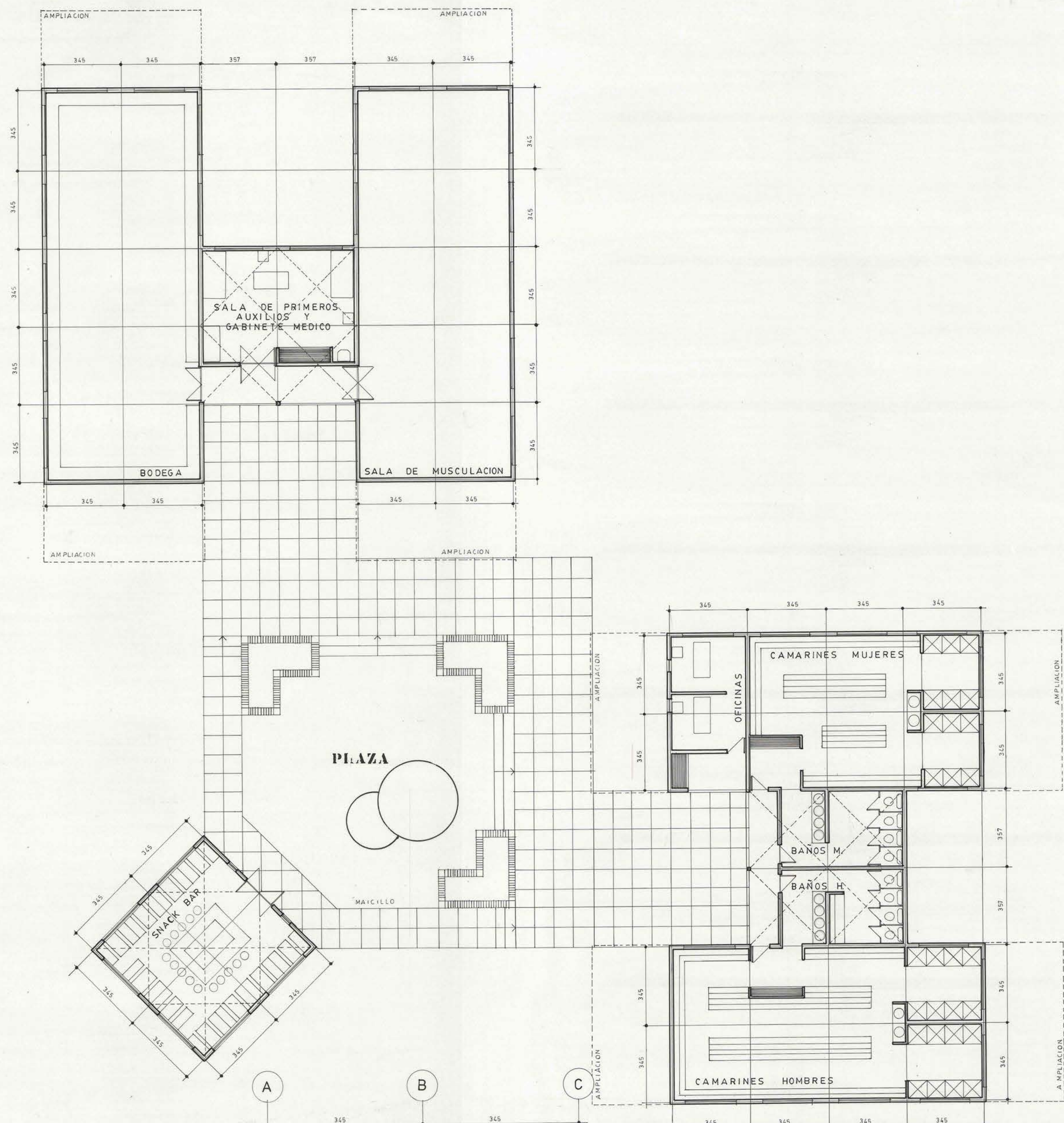
PLANTA CONJUNTO esc. 1/100
