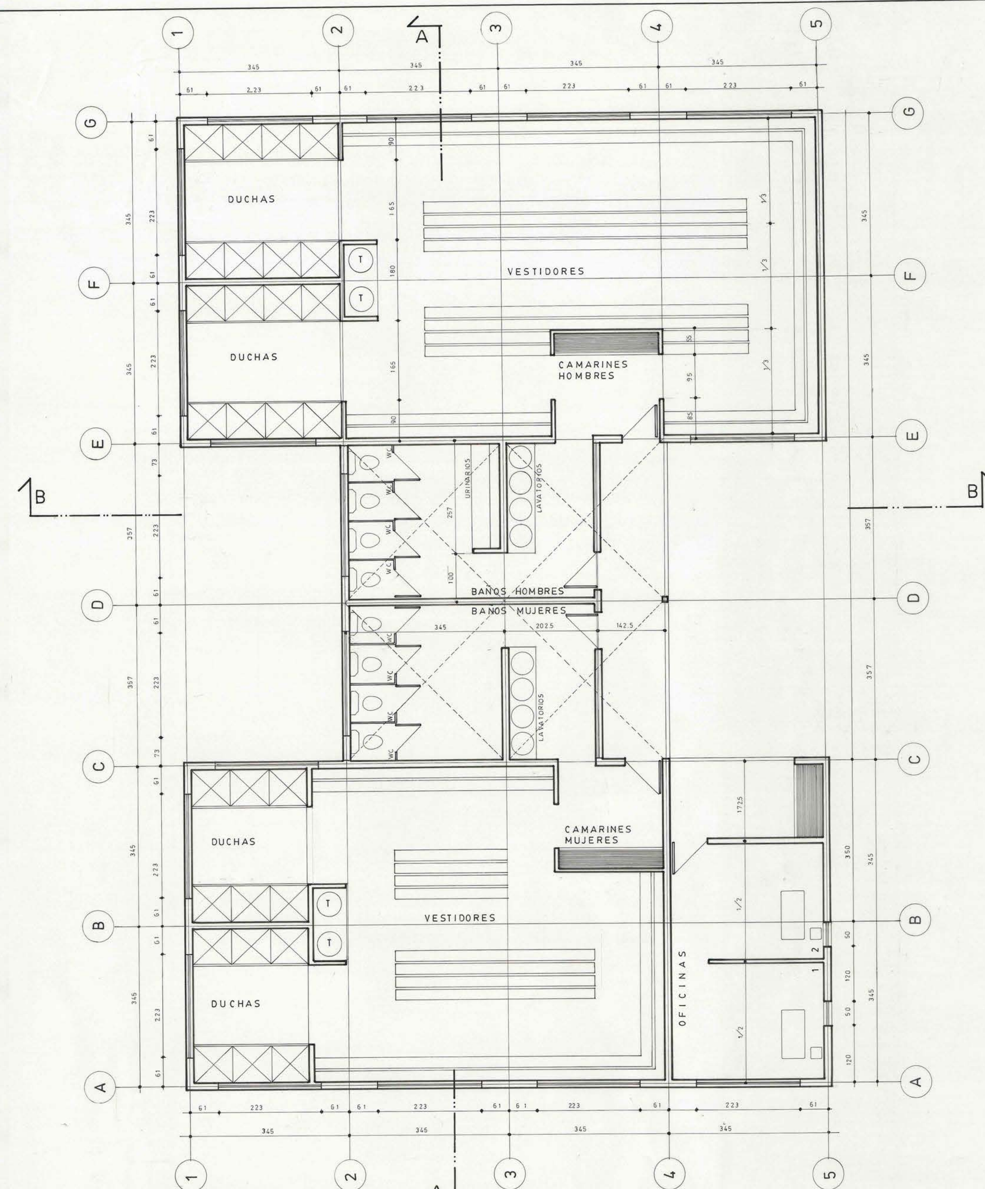
PLANTA CAMARINES esc. 1/50
