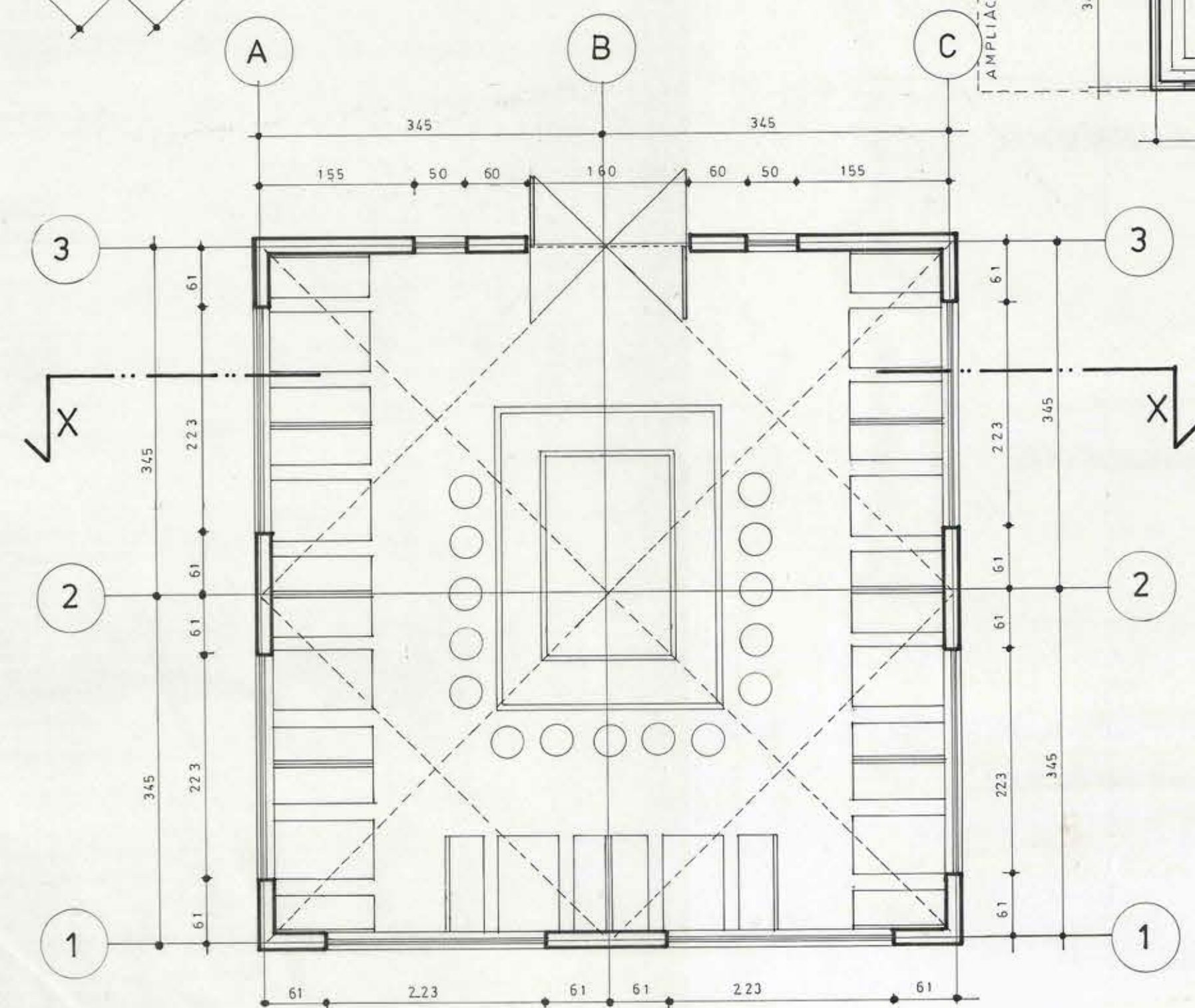
PLANTA SNACK BAR esc. 1/50
