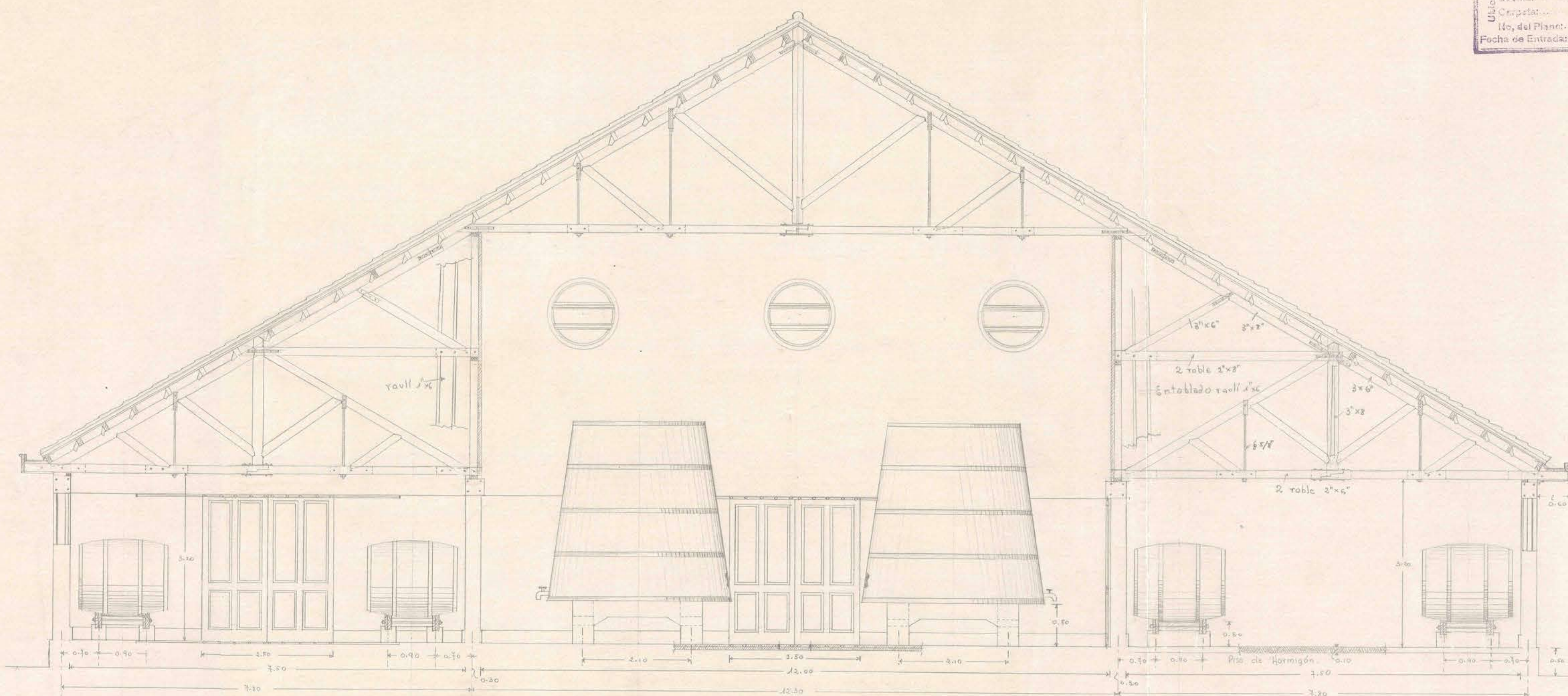
Sección a-b.
