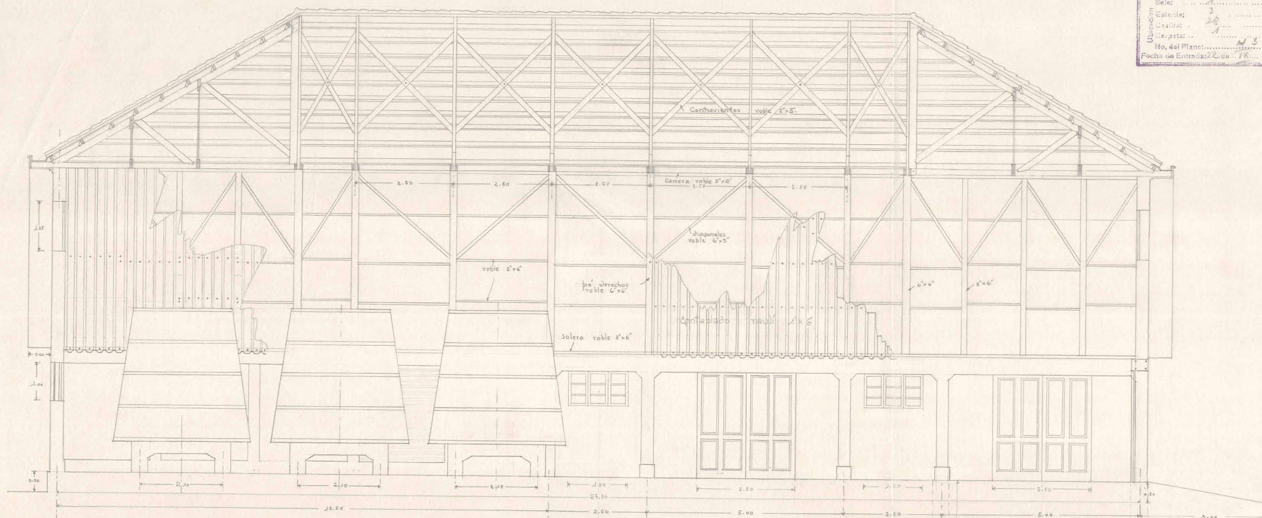
Sección C-d.
