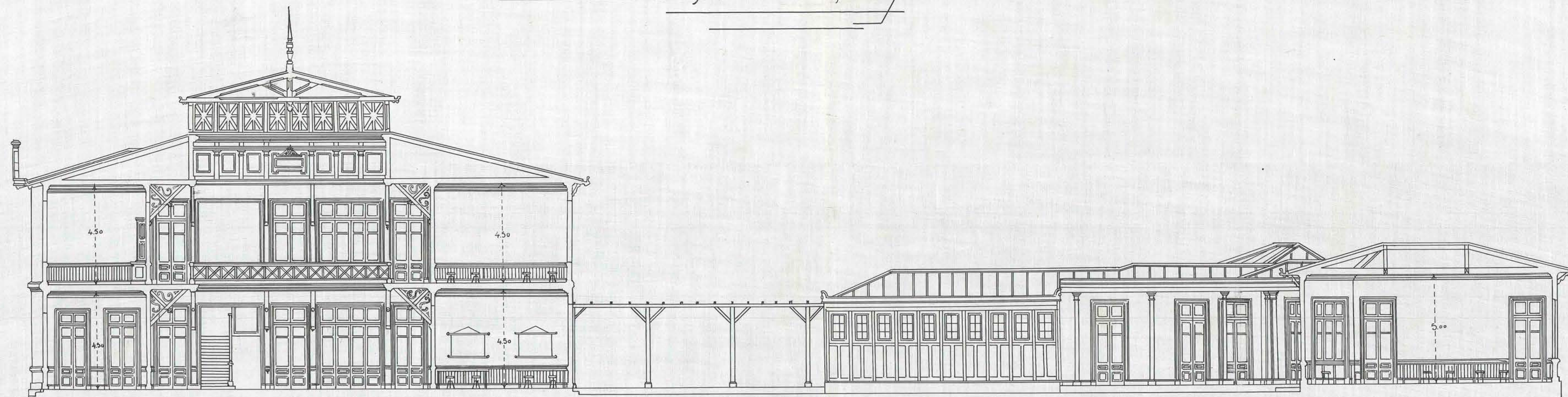
CORTE LONGITUDINAL
