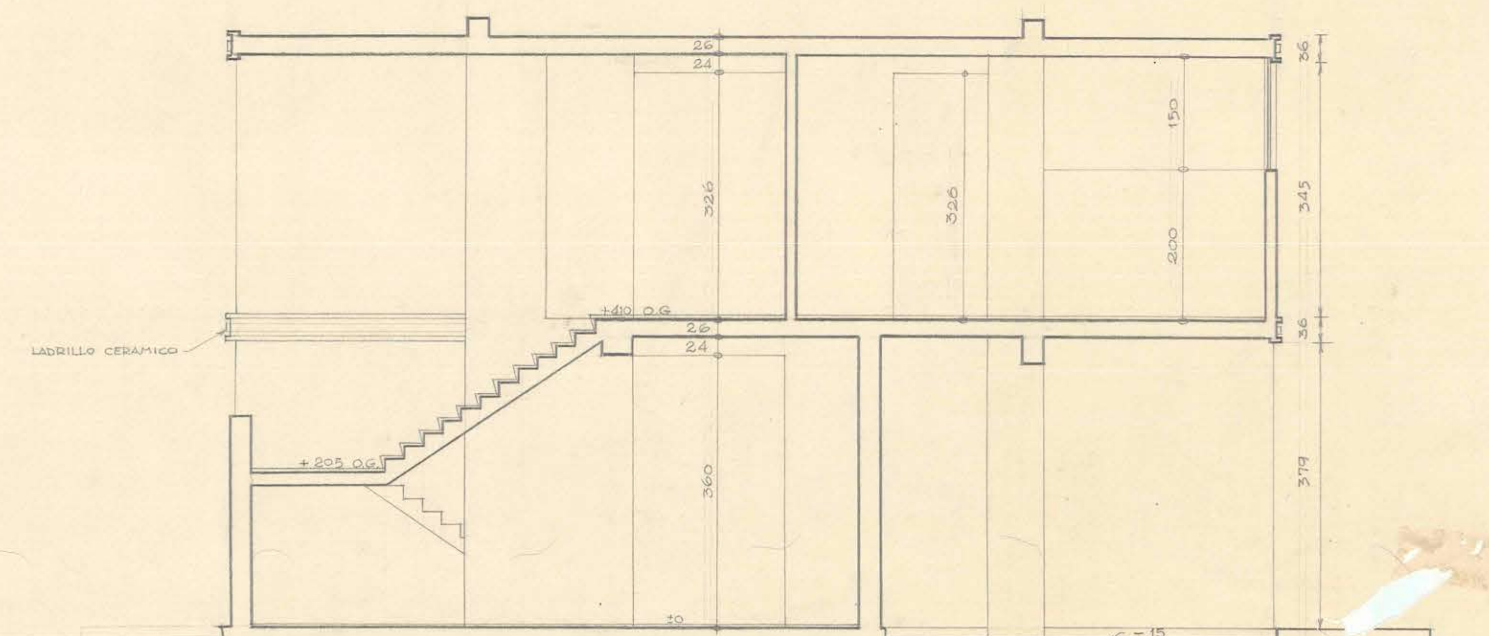
CORTE D-D'
