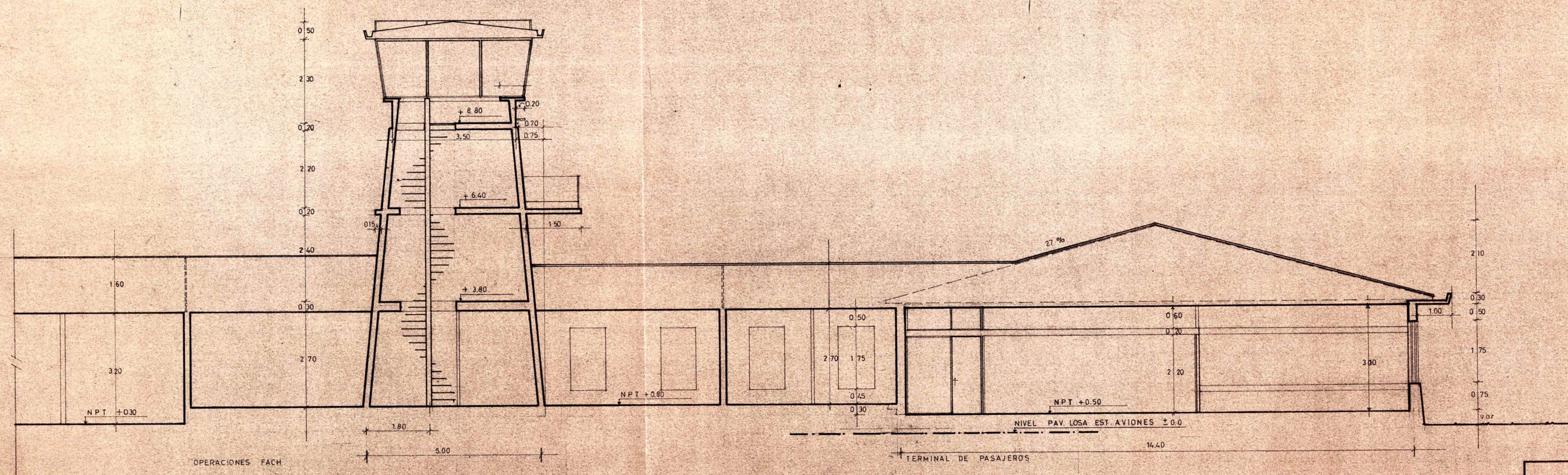
corte esquemático A-B
