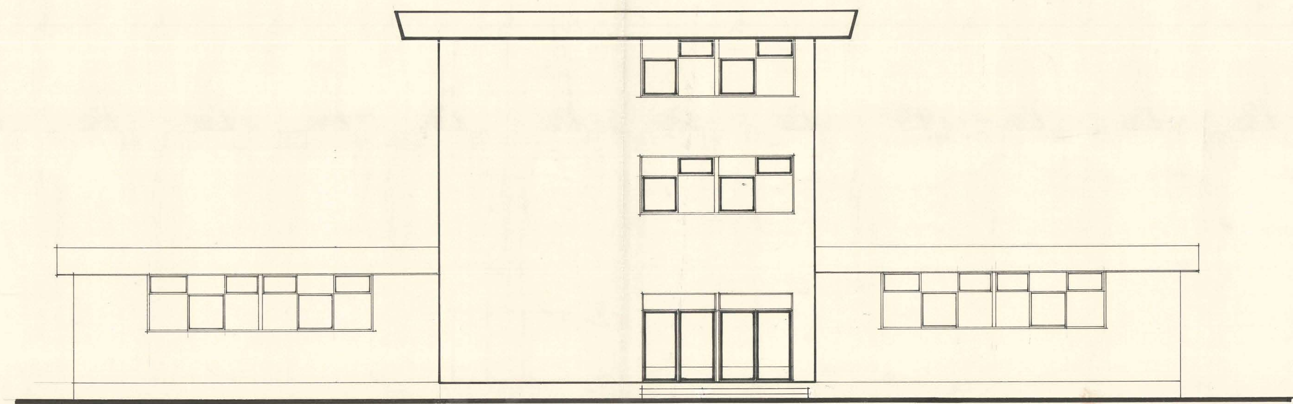
ELEV. NORTE
