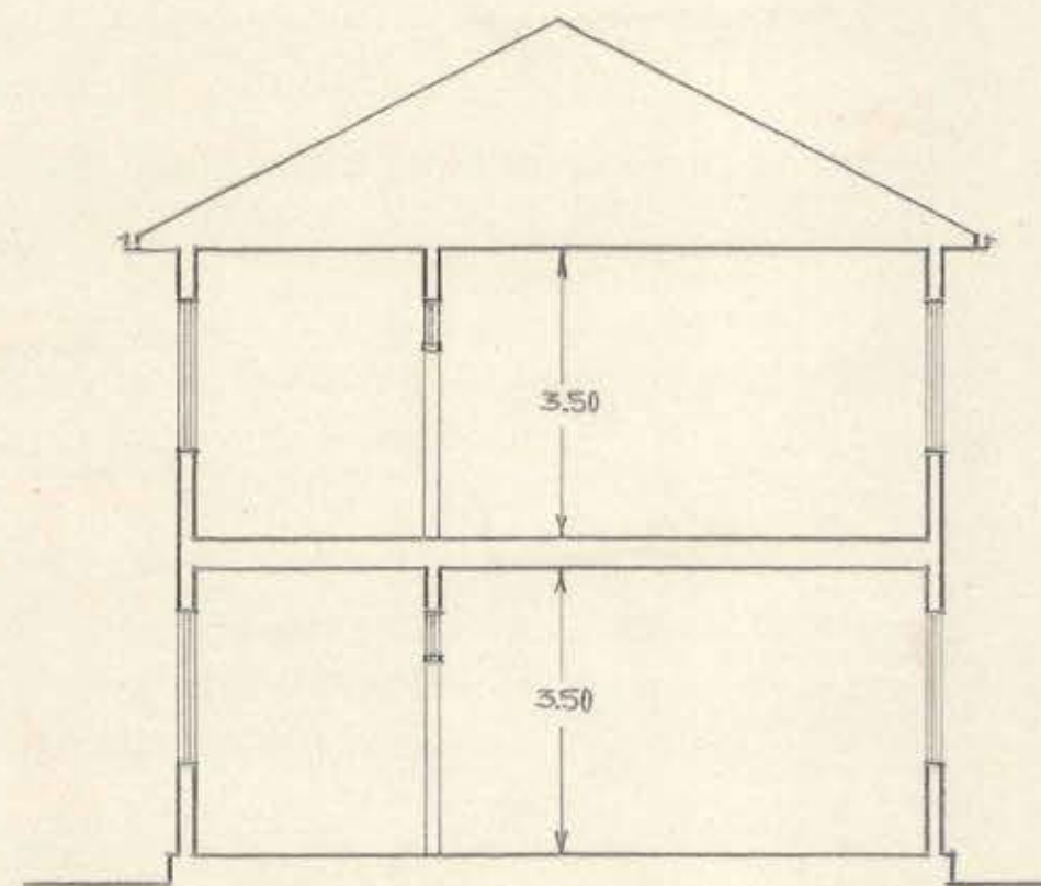
● CORTE A-B
