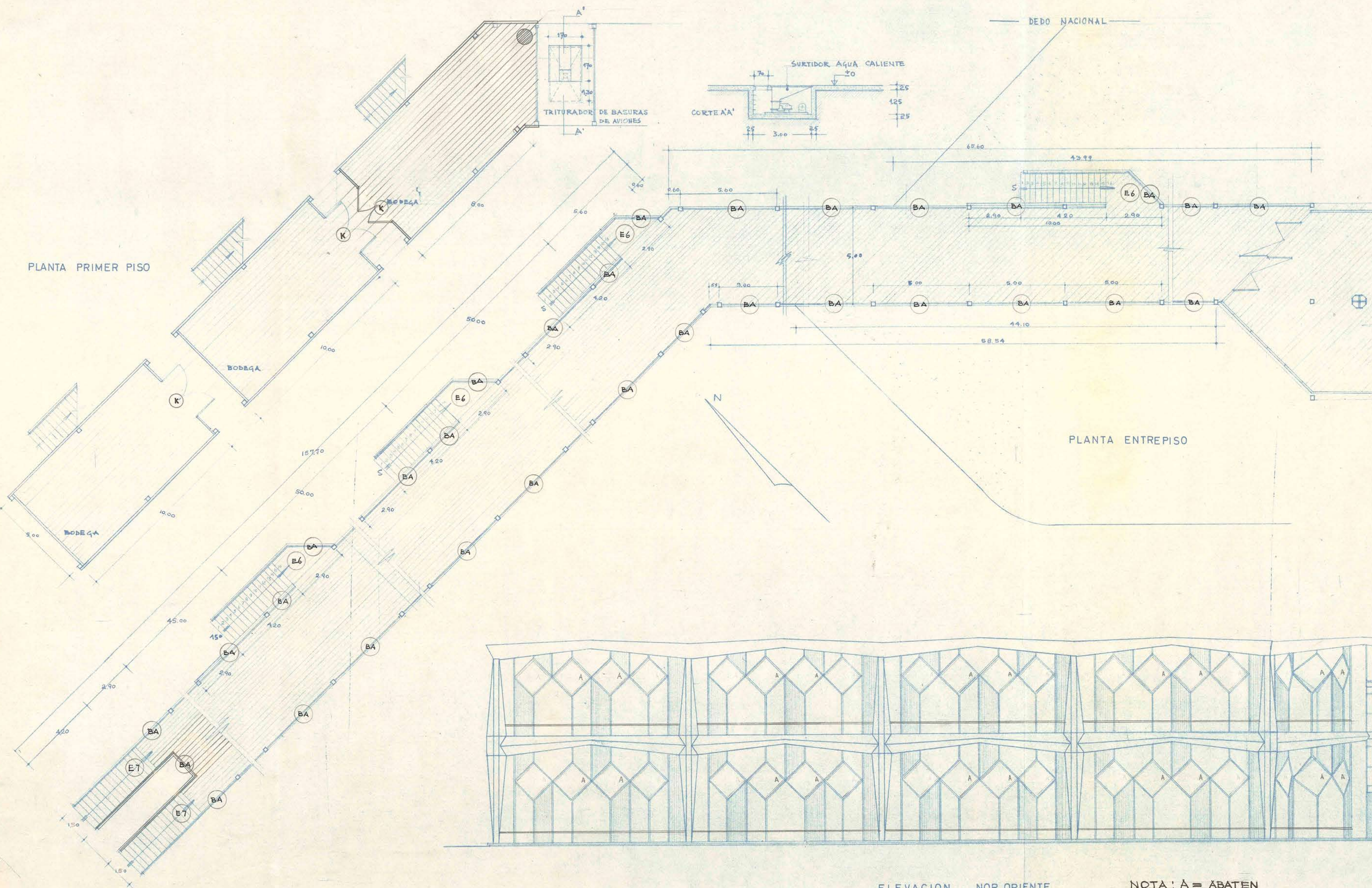
ELEVACION NOR ORIENTE
