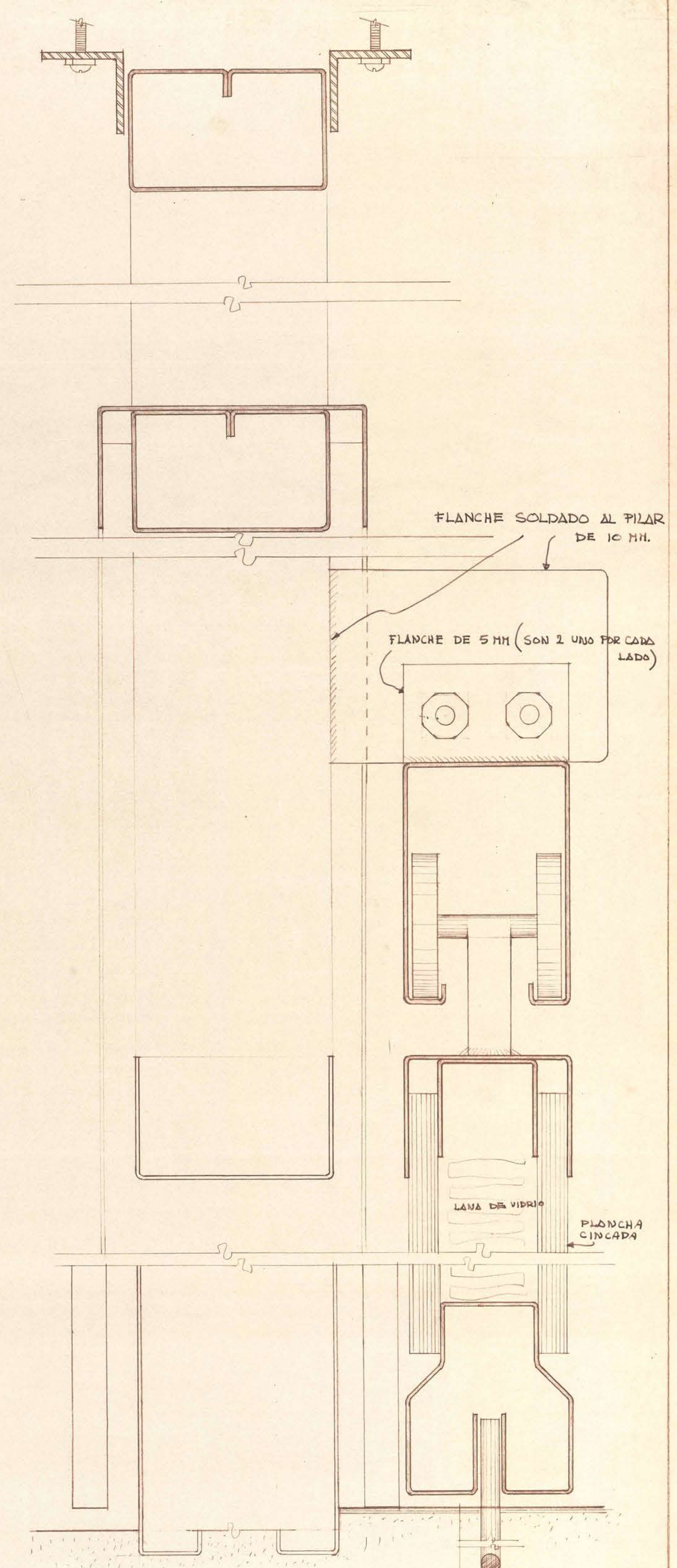
CORTE VERTICAL F-F' DE PUERTA CORREDERA
