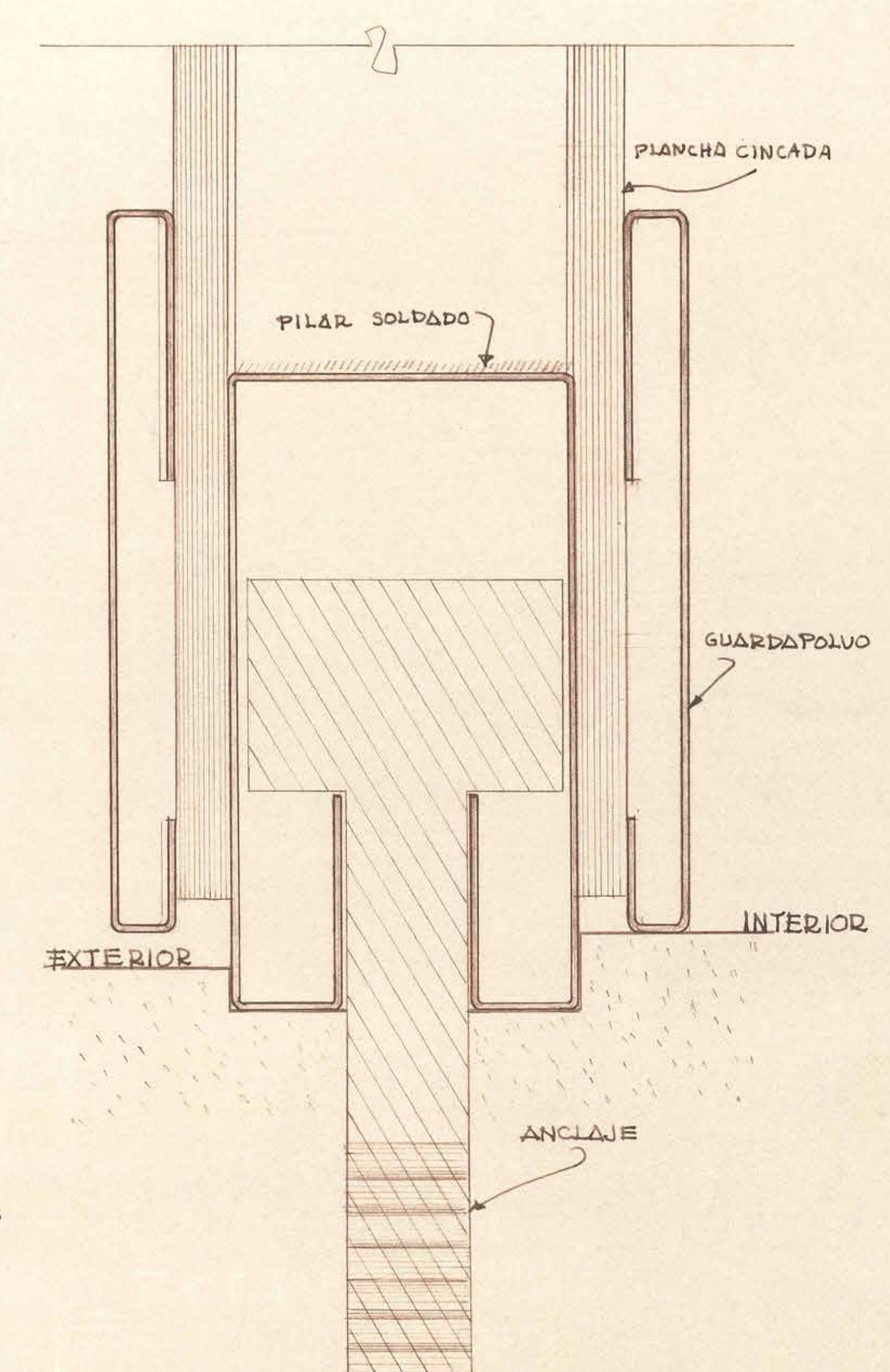
DETALLE TABIQUE EN SU PARTE INFERIOR ESC. NATURAL
