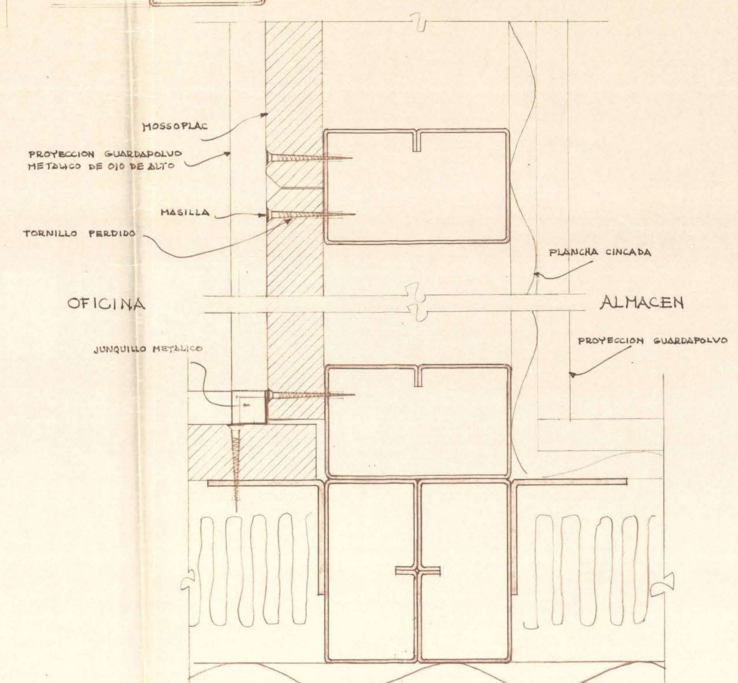
CORTE HORIZONTAL POR UN TABIQUE QUE SEPARA OFICINAS DE APODO DE LOS ALMACENES
