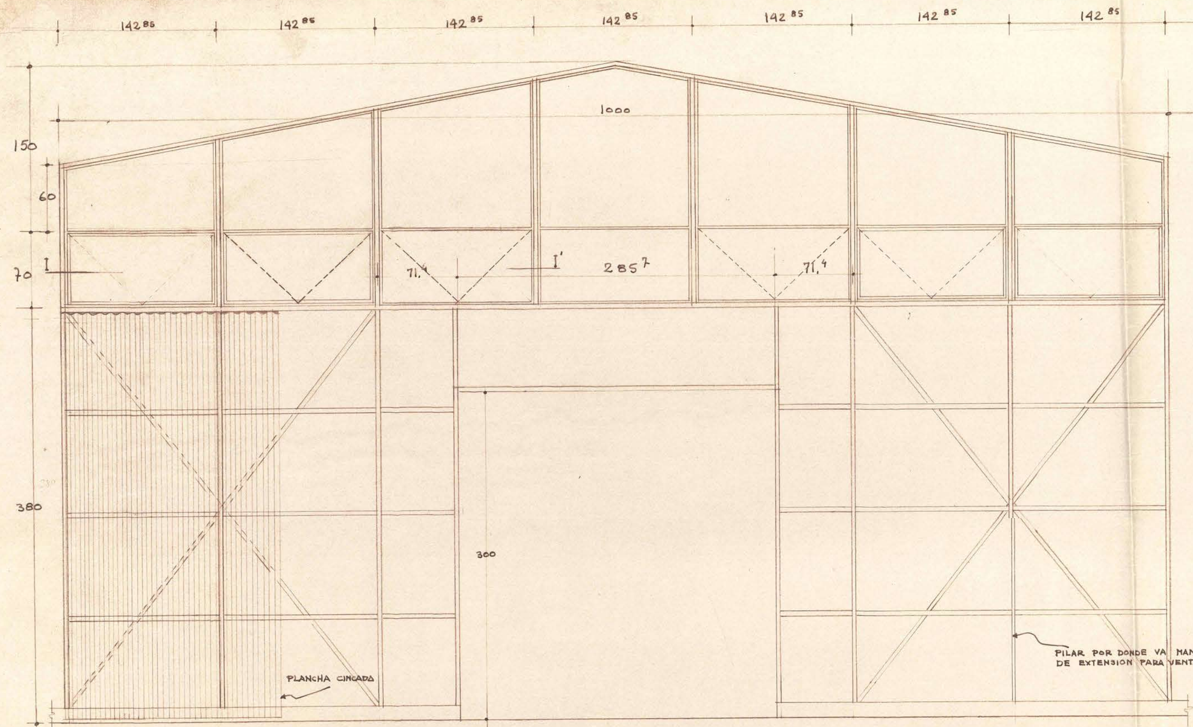
MODULO FACHADA EDIFICIO DE CARGA MOSTRANDO LA VENTANA SUPERIOR Y LA ESTRUCTURA
