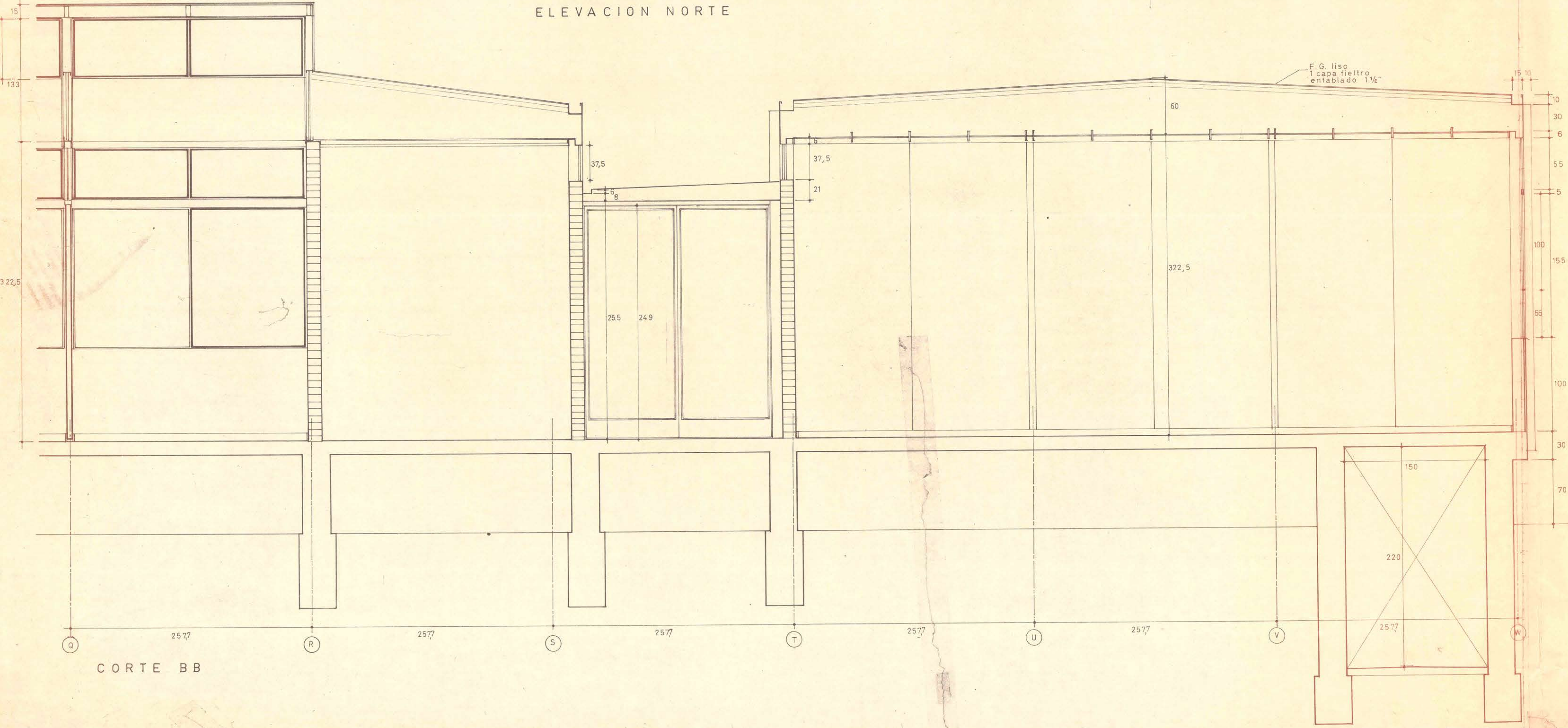
ELEVACION NORTE
