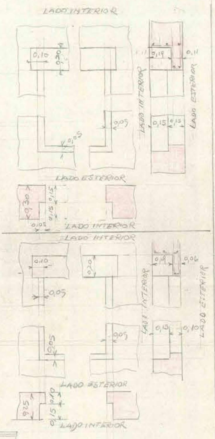
DETALLE VENTANAS 2º, 3º PISO
