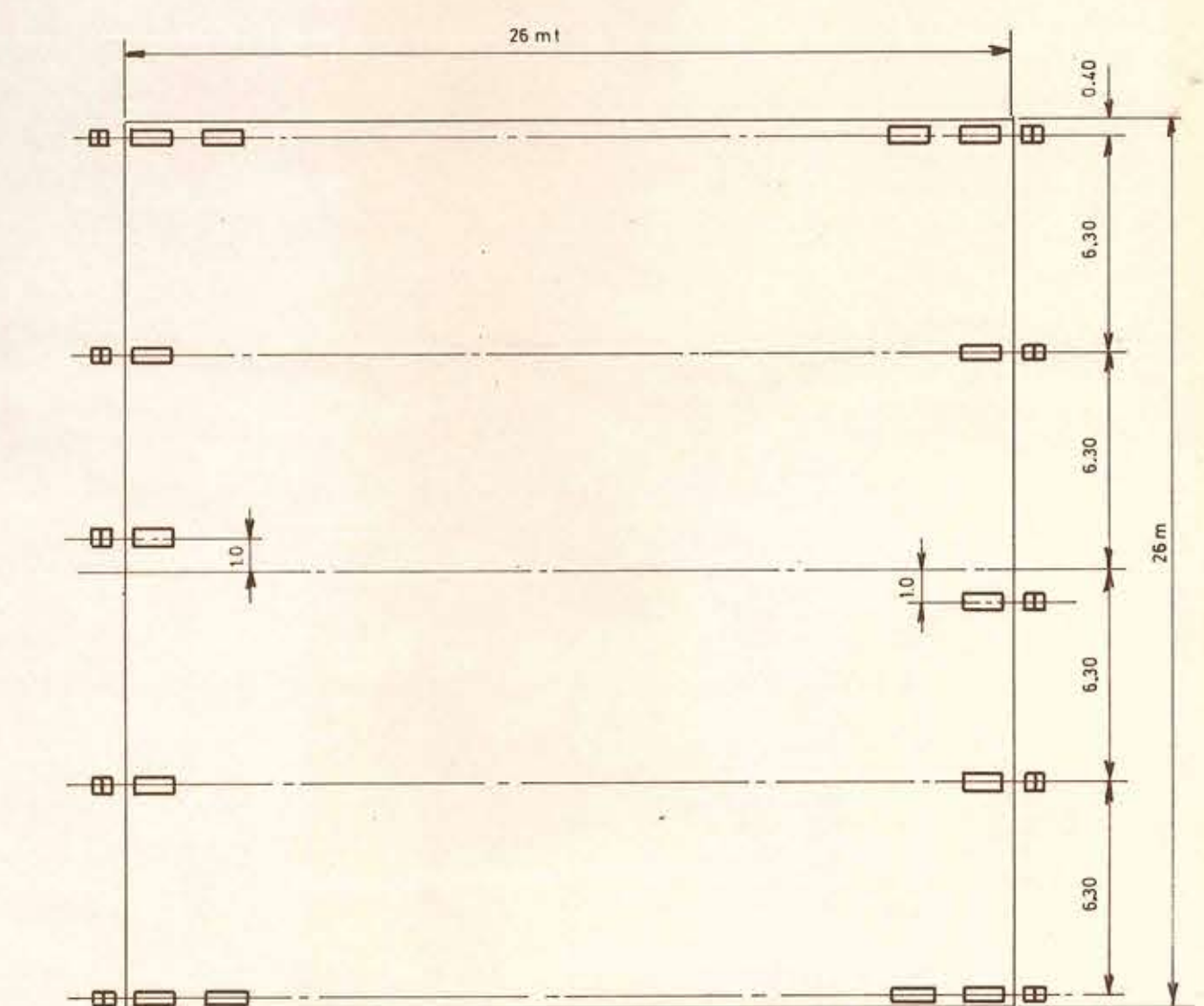
Ubicación de las columnas acústicas en la estereométrica
