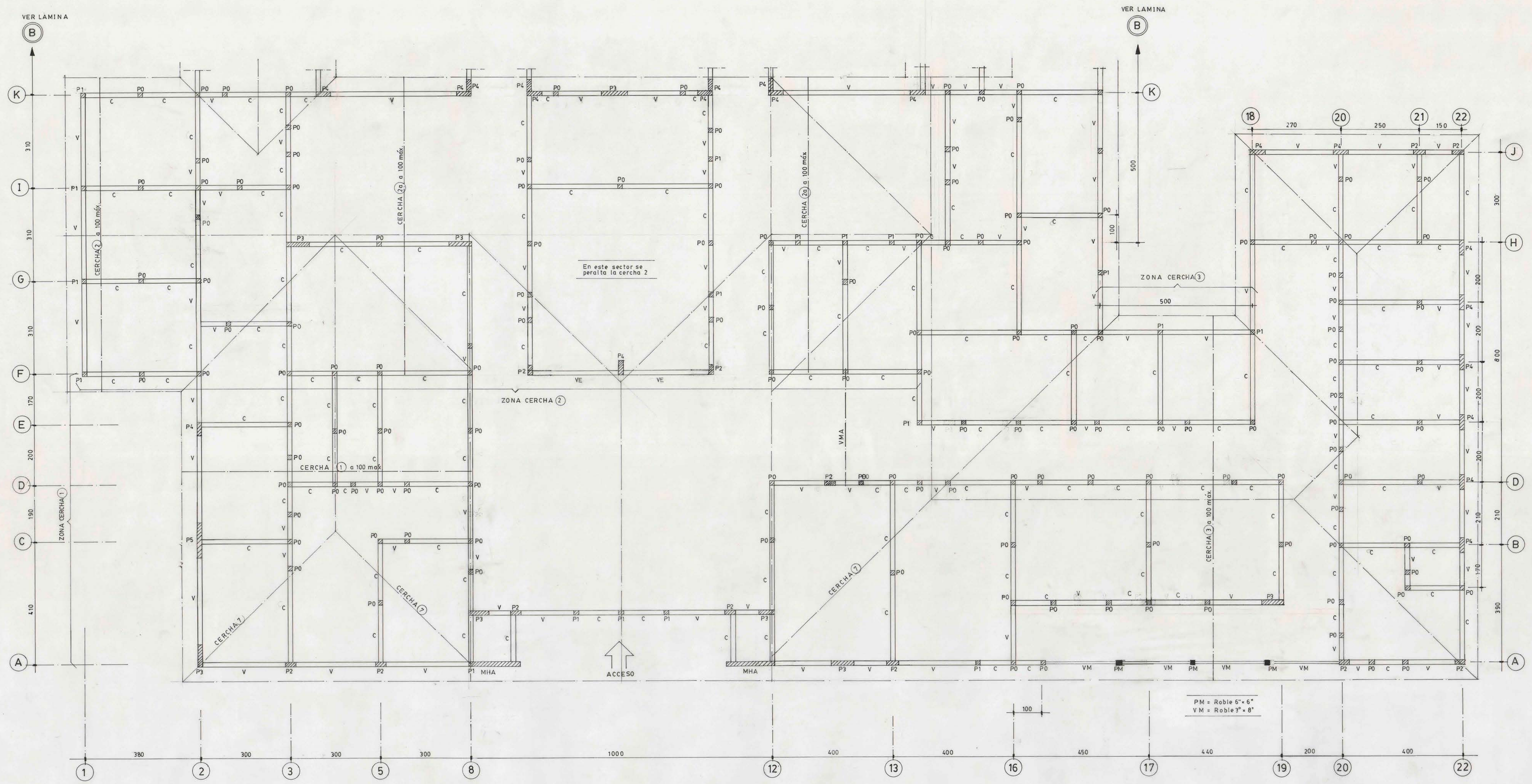
PLANTA ESTRUCTURA 1:50
