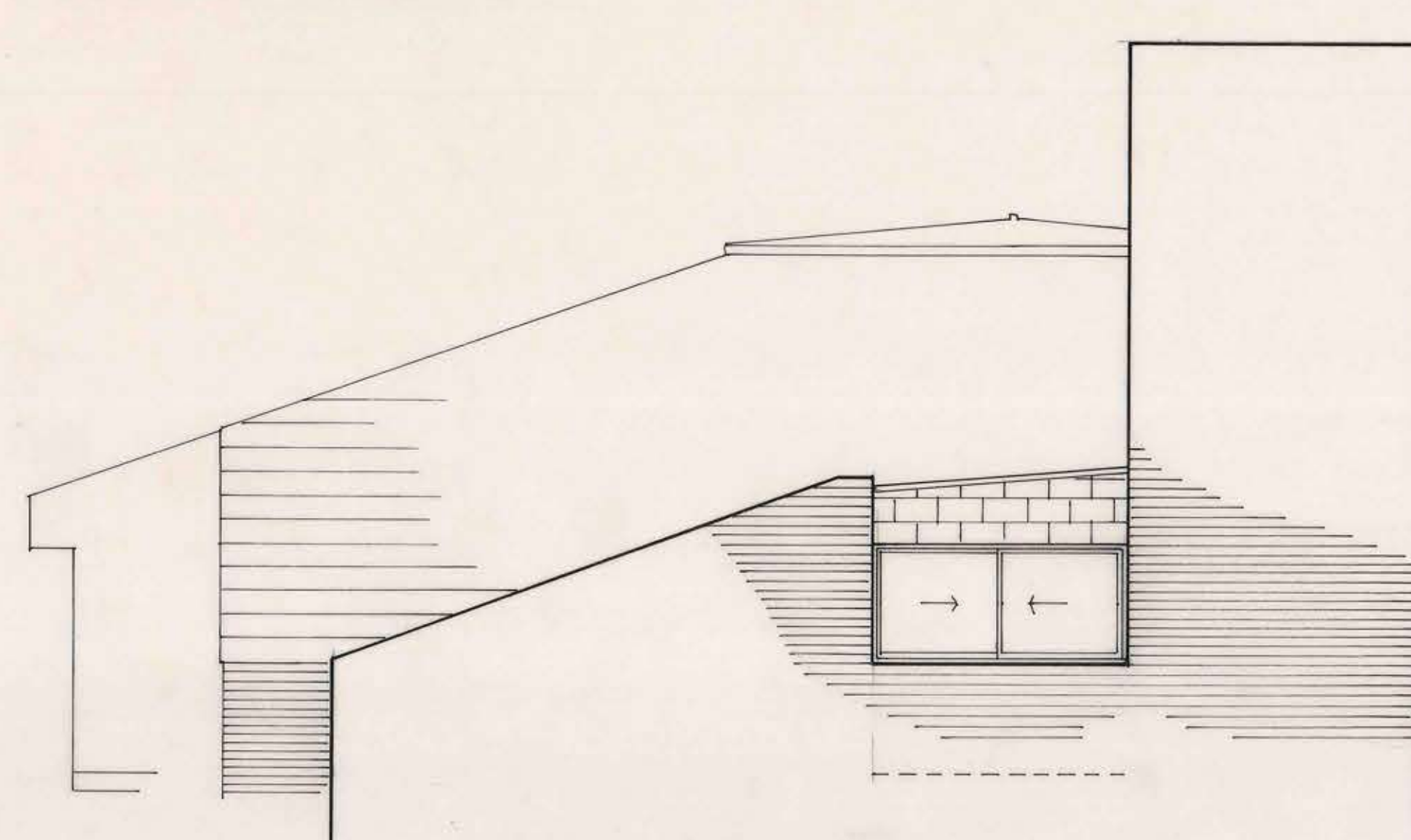
ELEVACION SUR
