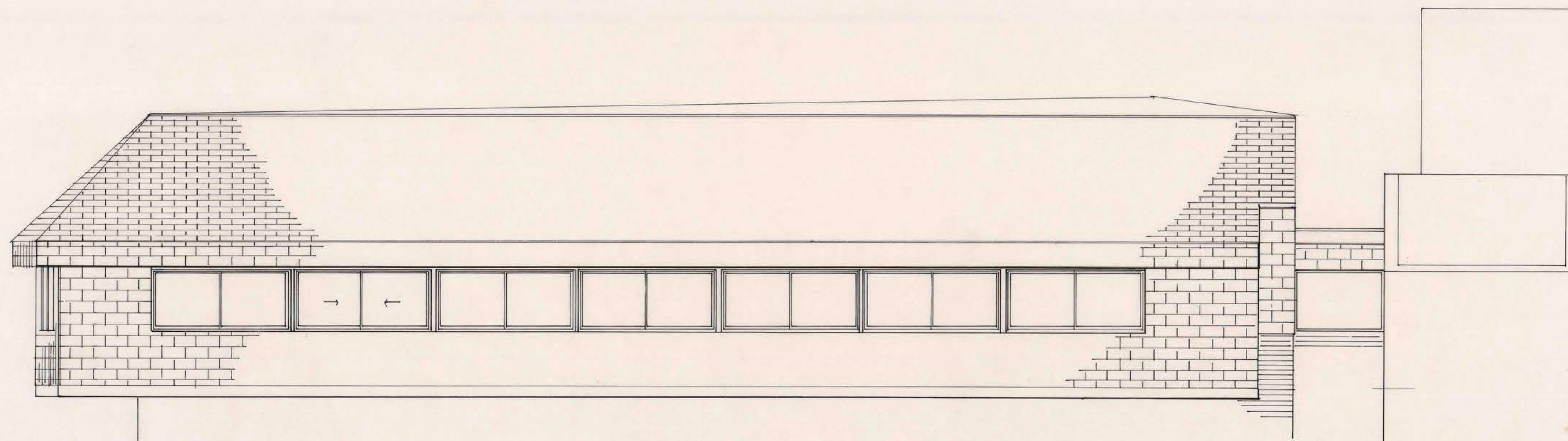
ELEVACION PONIENTE
