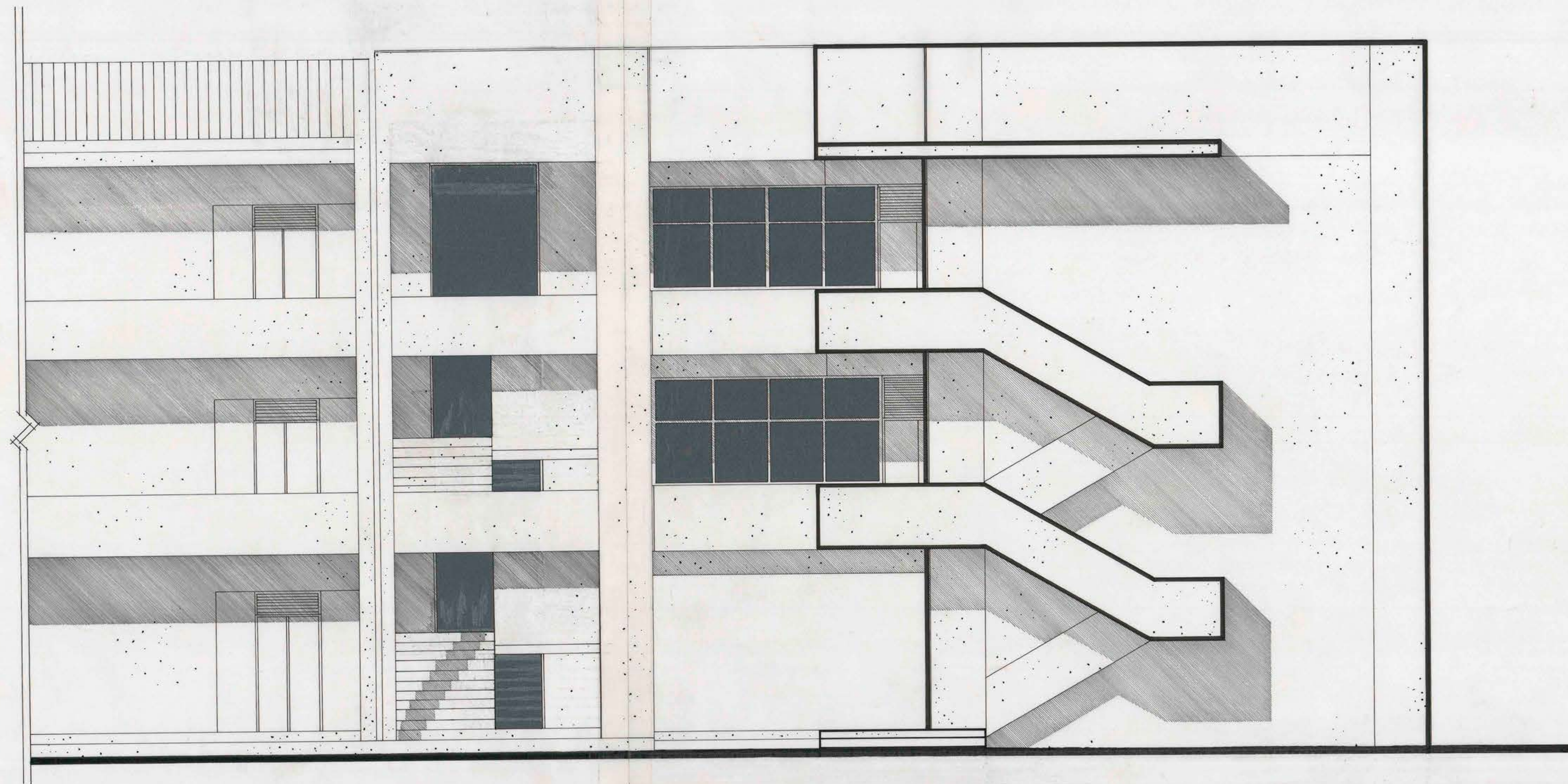
ELEVACION SUR escala 1: 50
