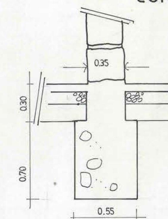
CORTE D D' 1:20
