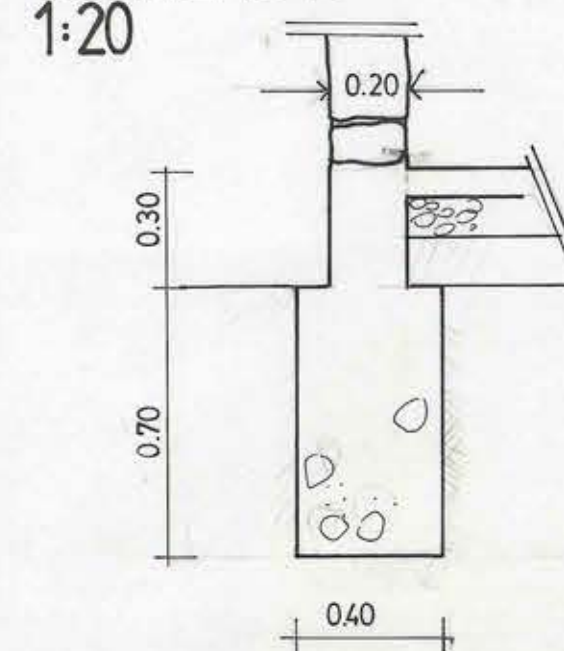
CORTE D D' 1:20
