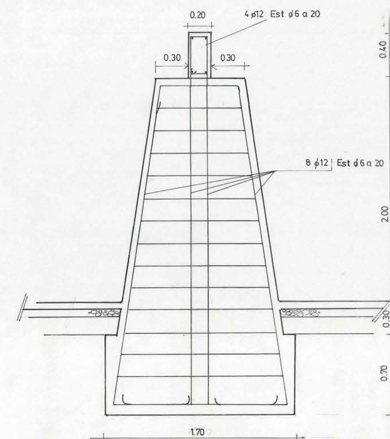
CORTE A A' 1:20
