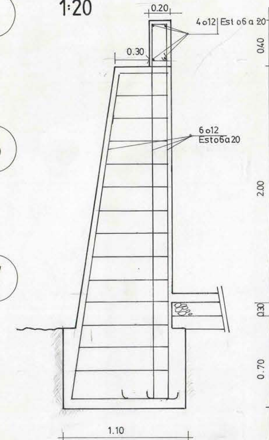
CORTE B B' 1:20
