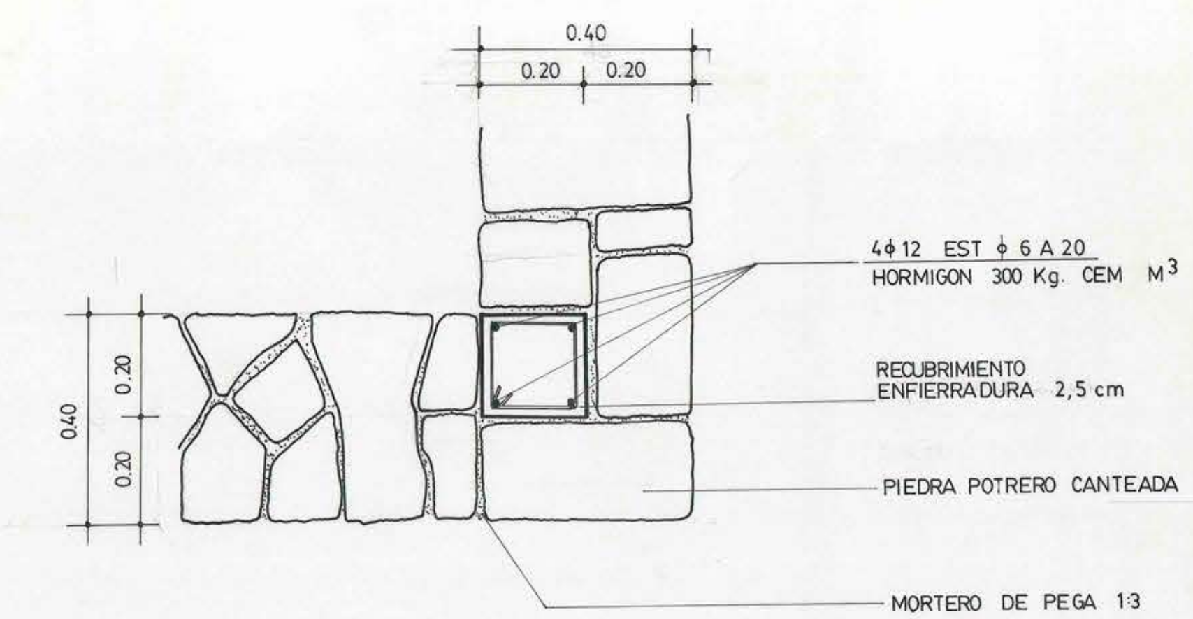
DETALLE PILAR ENCUENTRO MUROS Esc. 1:10
