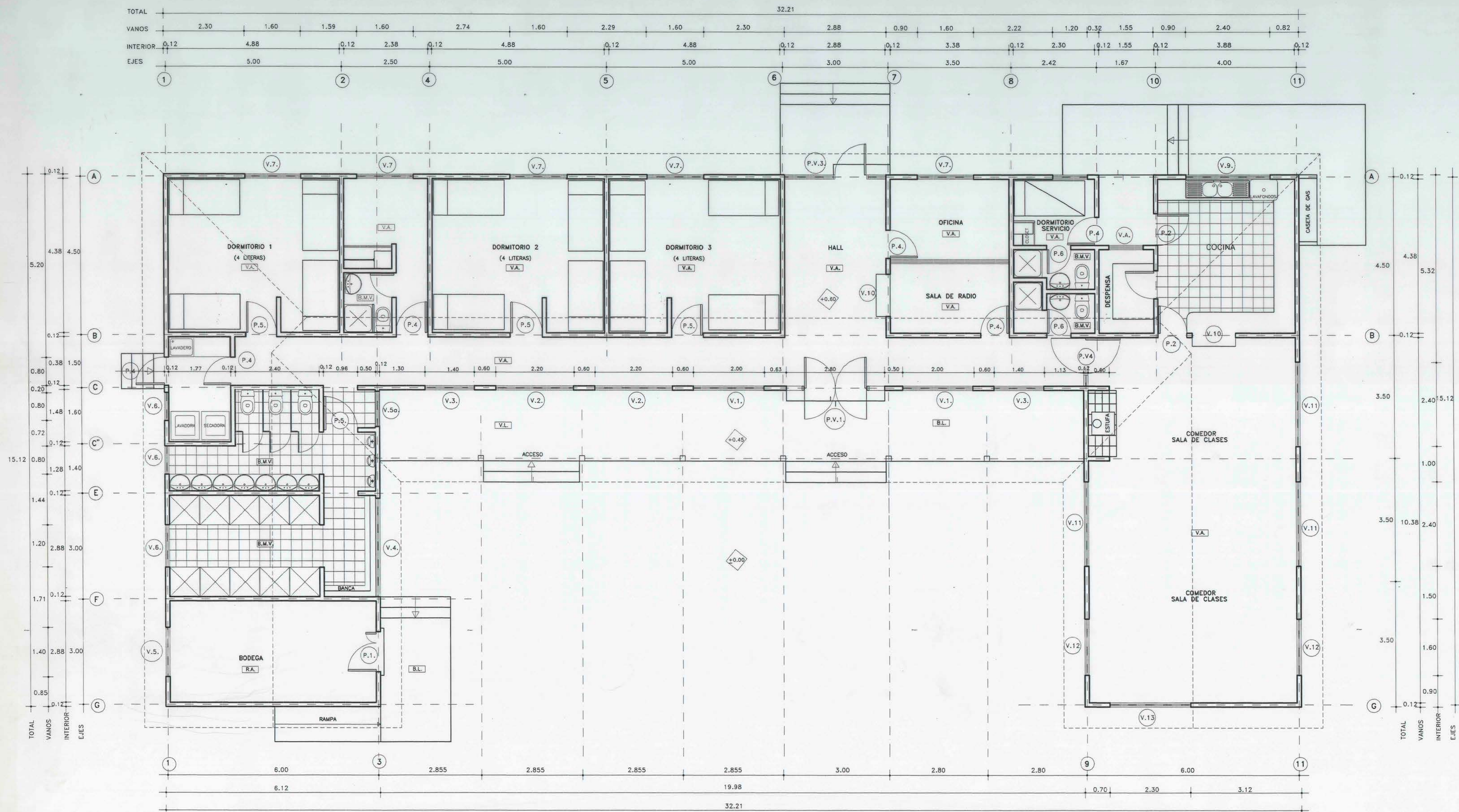
PLANTA ESCALA 1:50
