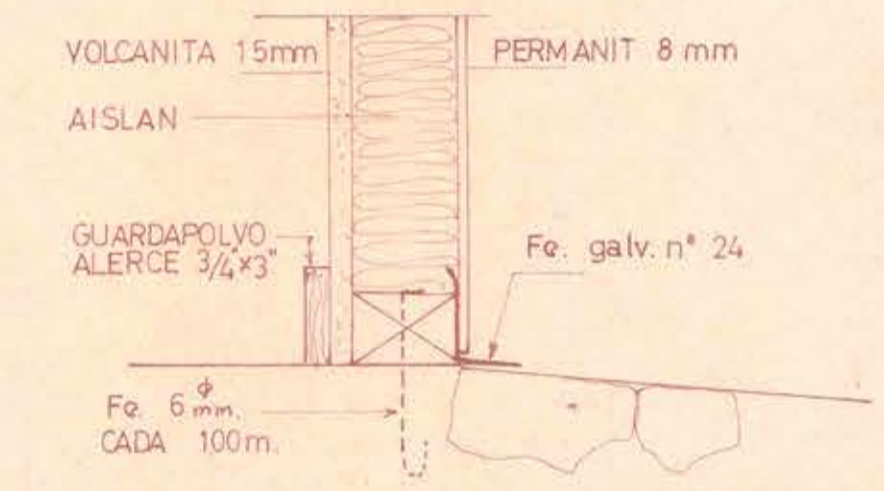
DET. C esc: 1:5
