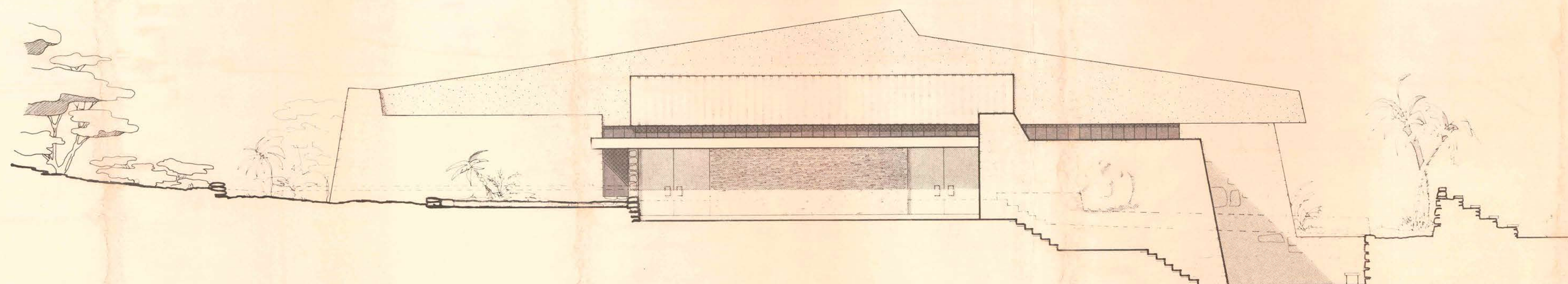
FACHADA NORTE E.S.C. 1/75
