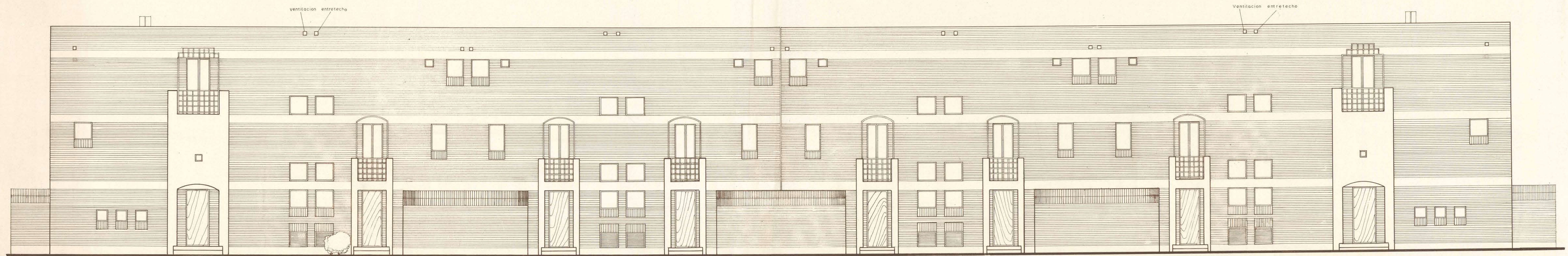
Elevación Sur
